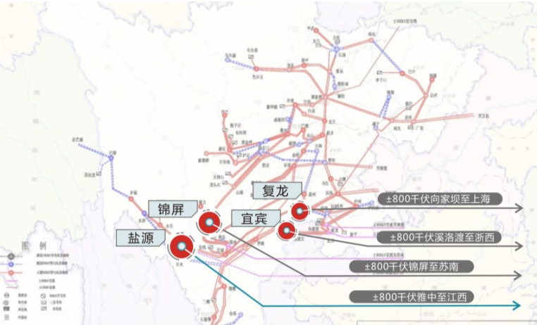
2020 年四川特高压电网目标网架
