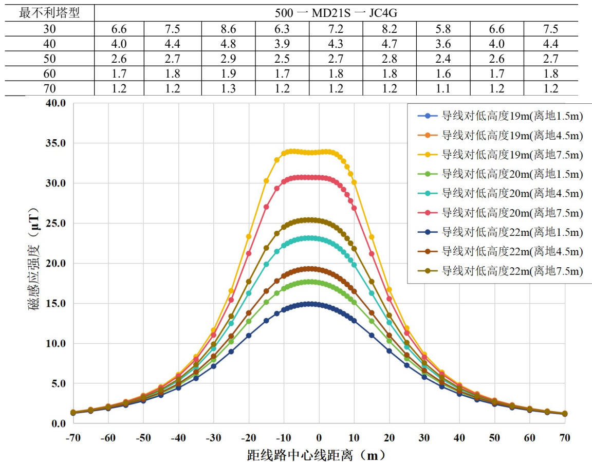
(续) 图 6-11 本段线路在民房等公众曝露区域最不利塔型磁感应强度随距离变化趋势图
