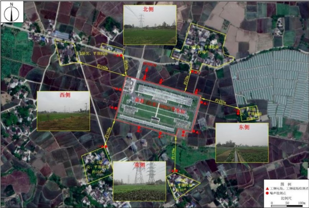
图 6-1 类比变电站的监测布点情况
