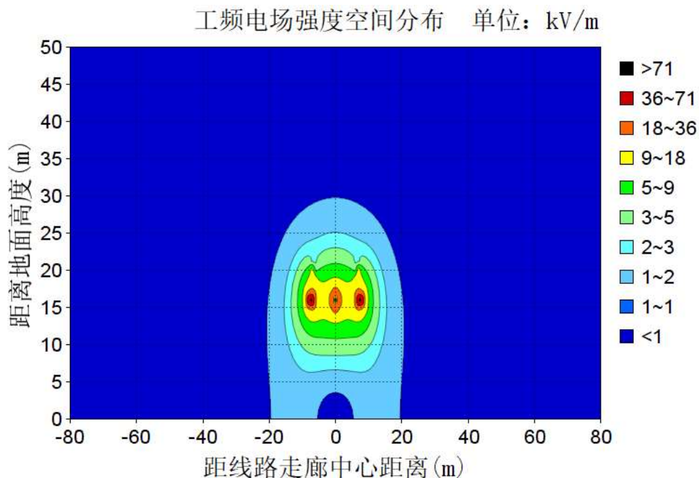
图 6-19 本段线路导线对地高度 16m 的电场强度等值线图
