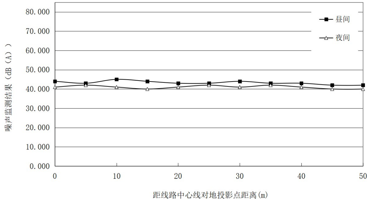
图 6-30 类比线路（500kV 谭邠一二线）噪声度随距中心线距离变化趋势图
