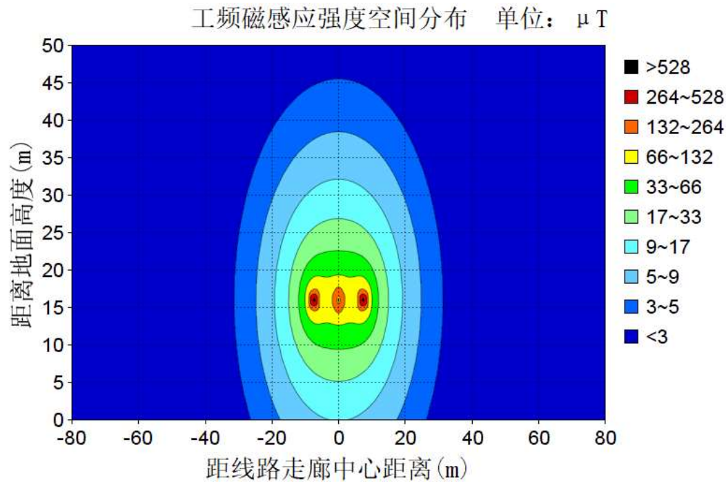
图 6-21 本段线路导线对地高度 16m 的磁感应强度等值线图
