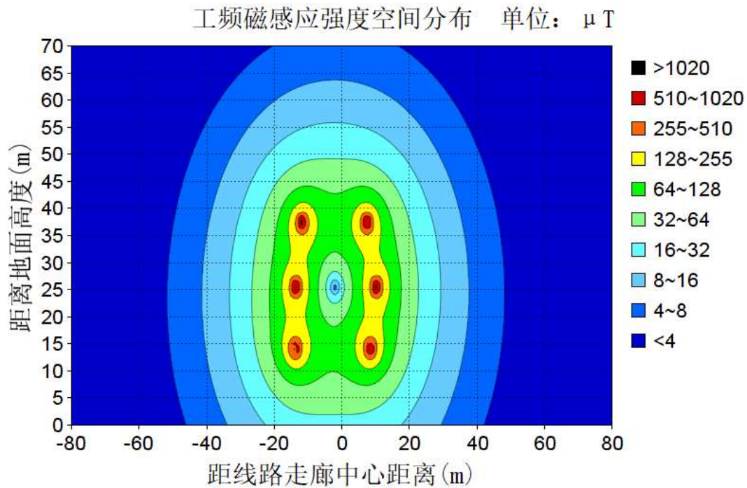
图 6-13 导线对地高度 14m 的磁感应强度等值线图
