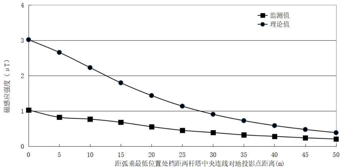
图 6-23 类比线路（瀑布沟电站-东坡I、II回）磁感应强度随距中心线距离变化趋势图
