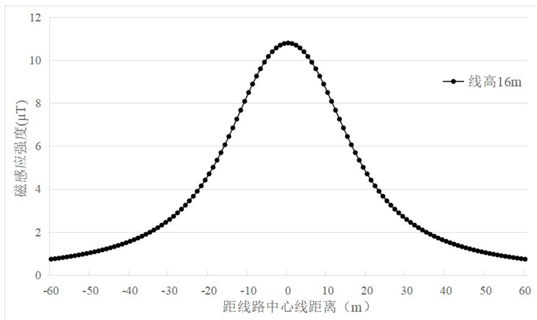
图 6-20 本段线路磁感应强度随距离变化趋势图
