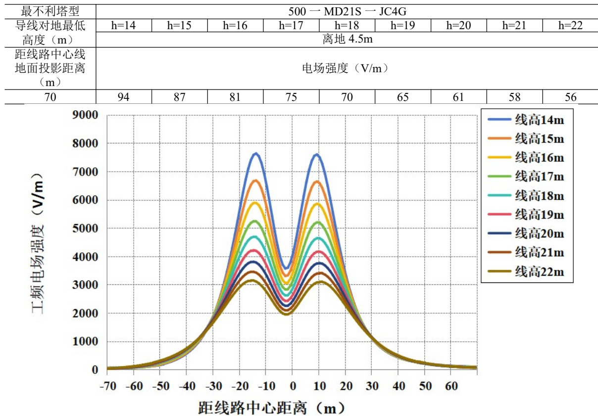
图 6-6 线路在公众曝露区电场强度随距离变化趋势图 (距地面 4.5m 高处)
