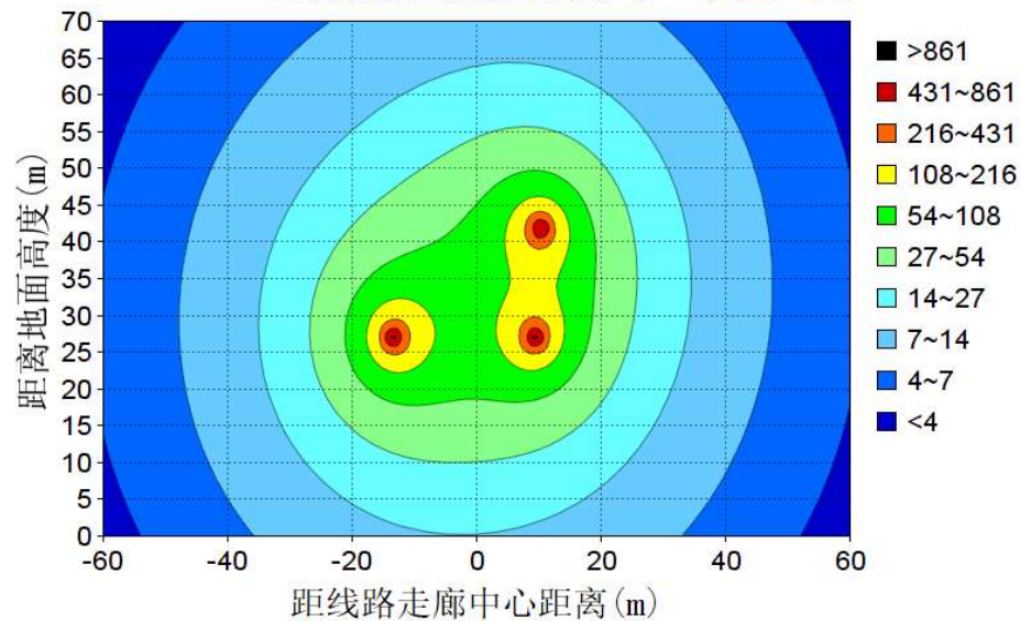
图 6-16 本线路磁感应强度随距离变化趋势图 工频磁感应强度空间分布 单位: \mu\text{T}
