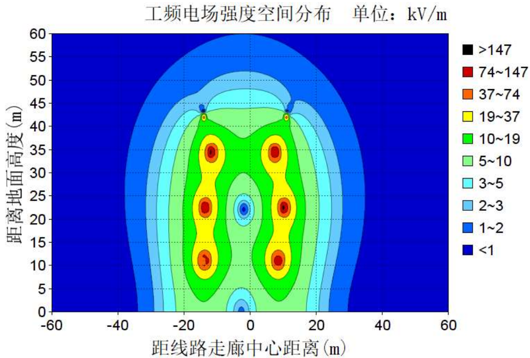
图 6-8 导线对地高度 11m 的电场强度等值线图 (单位: kV/m)
