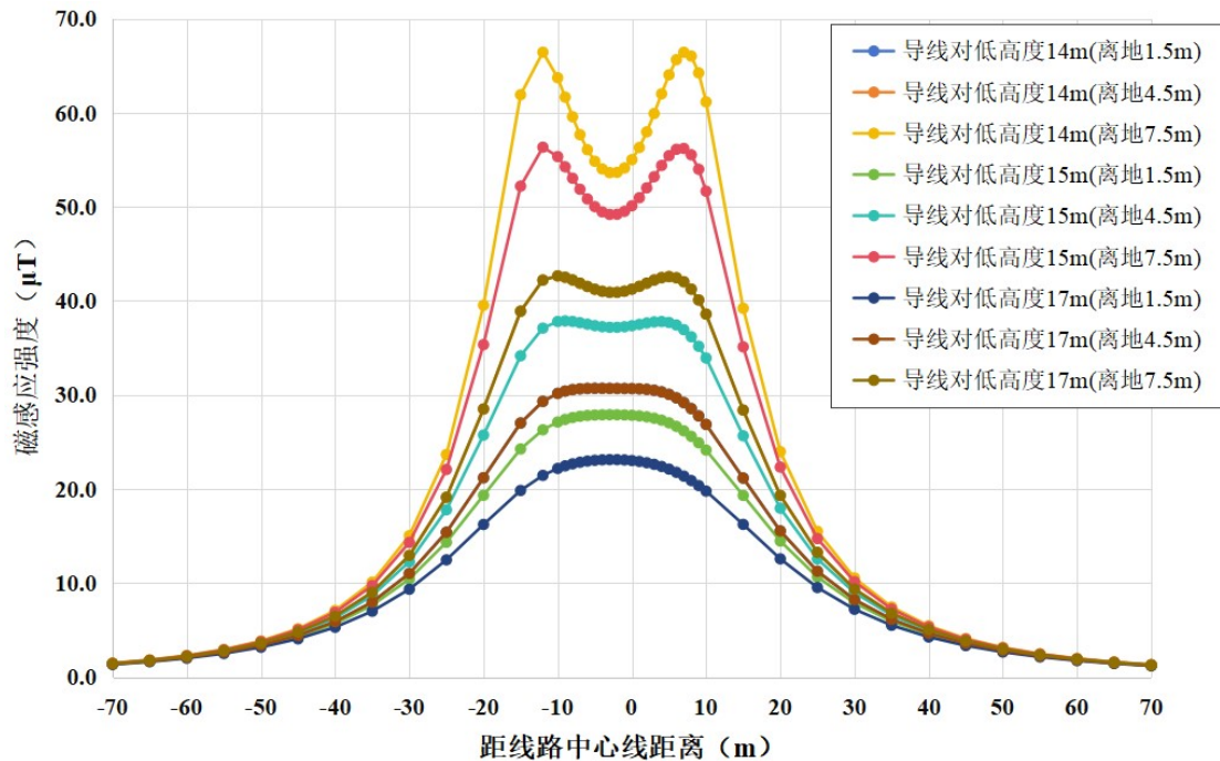
图 6-11 本段线路在民房等公众曝露区域最不利塔型磁感应强度随距离变化趋势图 (续) 表 6-19 本段线路在民房等公众曝露区域最不利塔型磁感应强度预测结果
