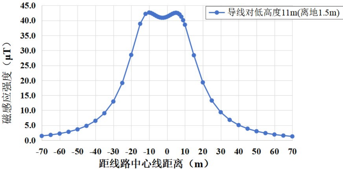
图 6-10 本段线路通过耕地、牧草地等场所最不利塔型磁感应强度随距离变化趋势图
