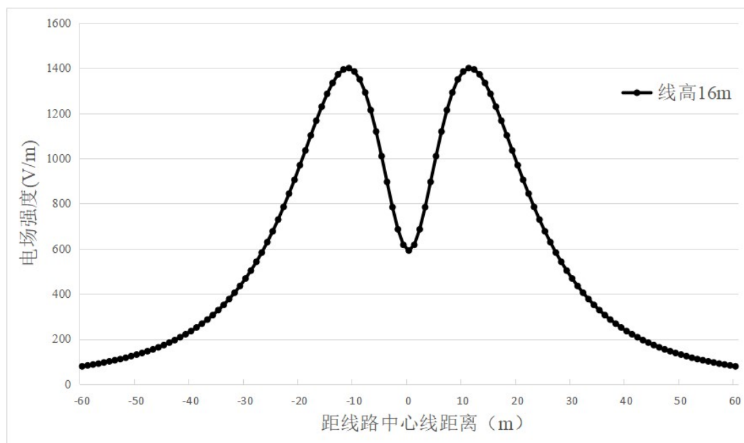
图 6-18 本段线路电场强度随距离变化趋势图
