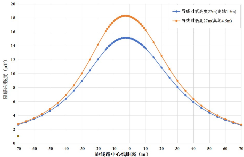
图 6-16 本线路磁感应强度随距离变化趋势图 工频磁感应强度空间分布 单位: \mu\text{T}
