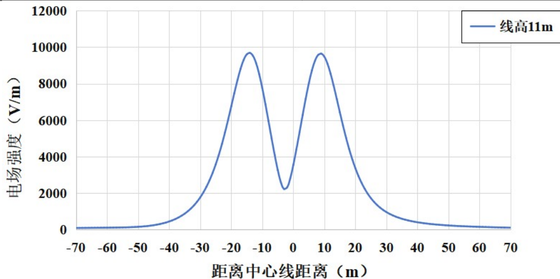
图 6-4 本段线路通过耕地、园地等场所最不利塔型电场强度随距离变化趋势图 表 6-14 本段线路在公众暴露区最不利塔型电场强度预测结果 (距地面 1.5m 高处)
