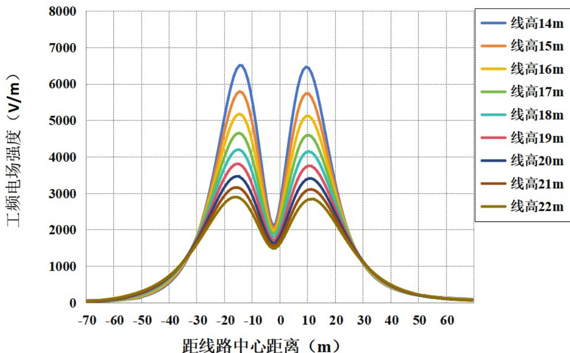
图 6-5 线路在公众暴露区电场强度随距离变化趋势图 (距地面 1.5m 高处)
