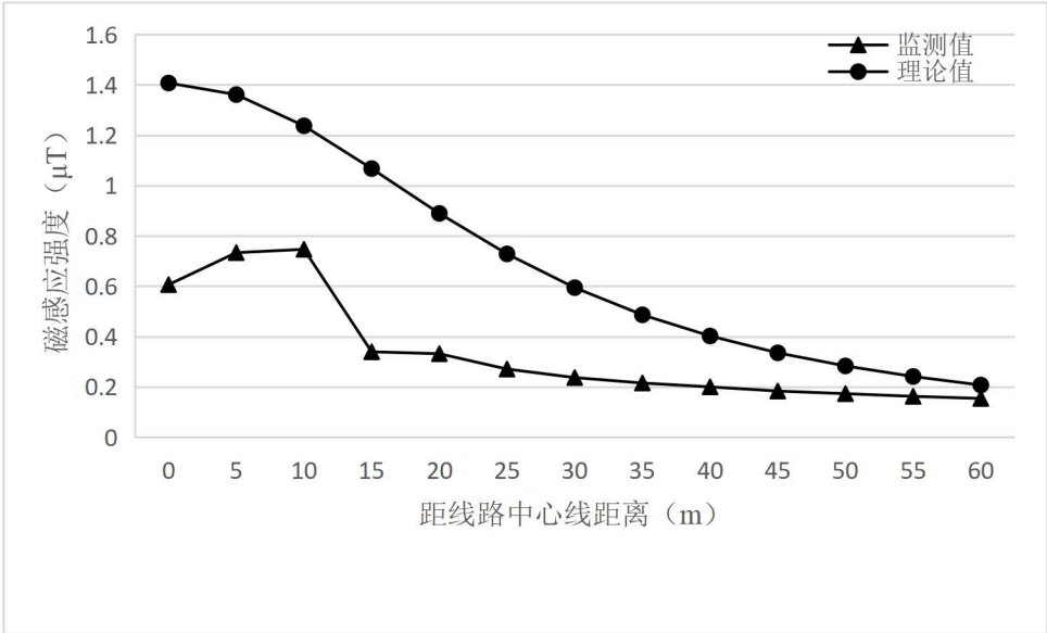
图 6-25 类比线路（220kV 江林线）磁感应强度随距中心线距离变化趋势图
