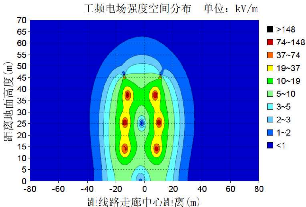
图 6-9 导线对地高度 14m 的电场强度等值线图 (单位: kV/m)
