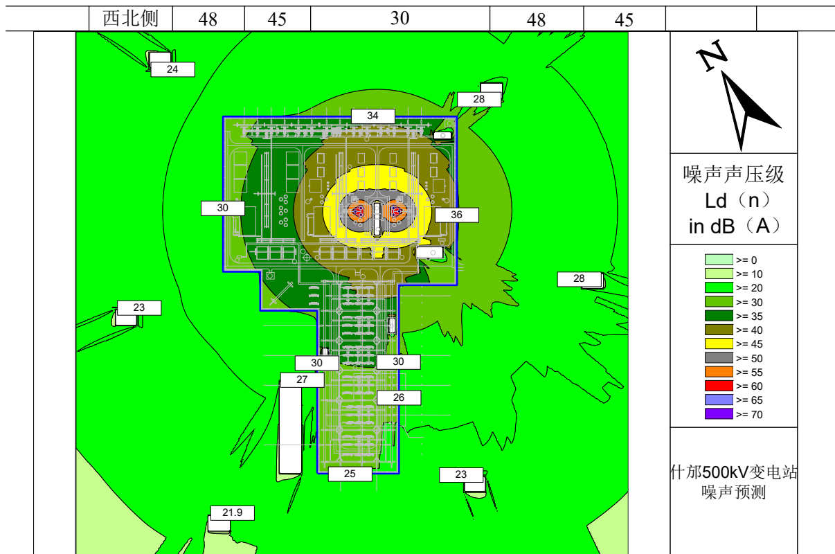
图 6-29 什邡变电站噪声预测（贡献值）等声级线图
