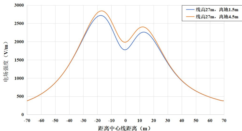
图 6-14 本段线路电场强度随距离变化趋势图
