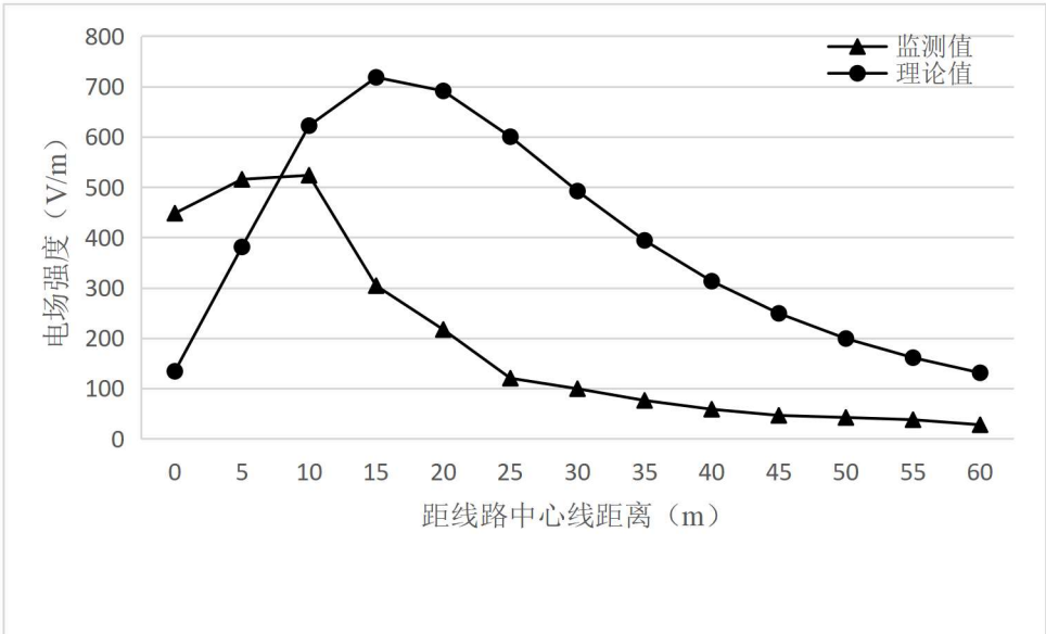
图 6-26 类比线路（220kV 江林线）电场强度随距中心线距离变化趋势图
