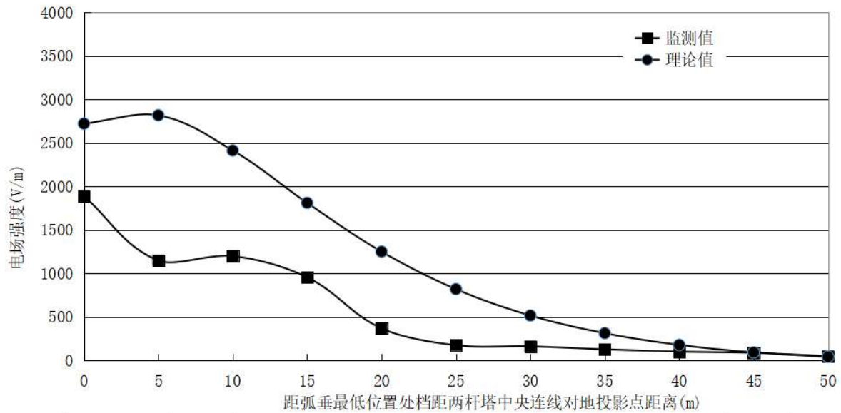
图 6-22 类比线路（瀑布沟电站-东坡I、II回）电场强度随距中心线距离变化趋势图
