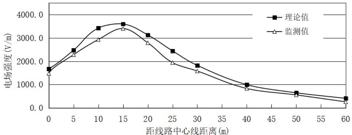
图 6-24 类比线路（500kV 洪板二线）电场强度随距中心线距离变化趋势图
