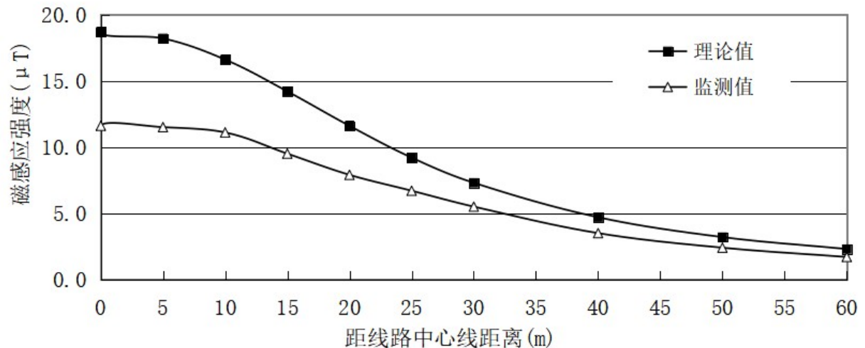
图 6-23 类比线路（500kV 洪板二线）磁感应强度随距中心线距离变化趋势图
