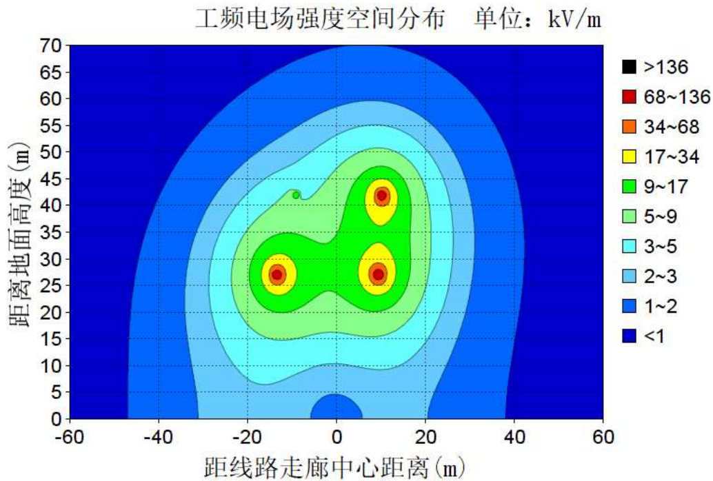
图 6-15 本段线路导线对地高度 27m 的电场强度等值线图
