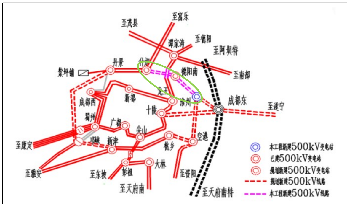
图 3-6 立体双环网构架示意图
