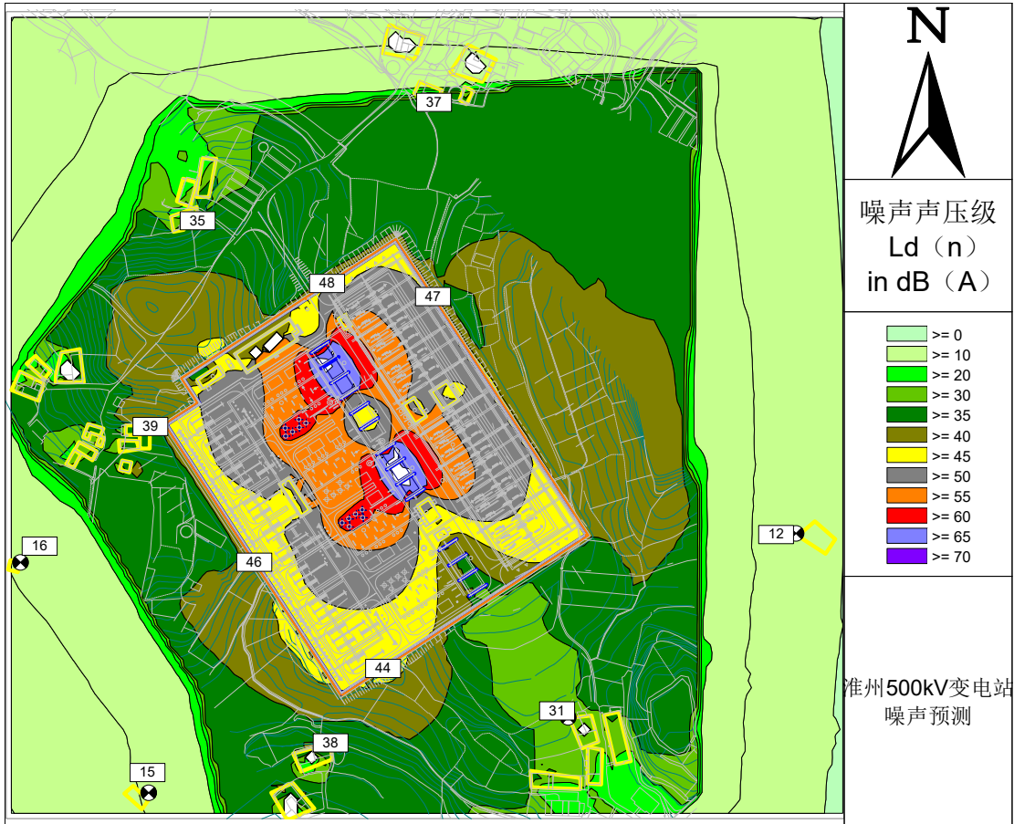
图 6-28 淮州变电站噪声预测（贡献值）等声级线图
