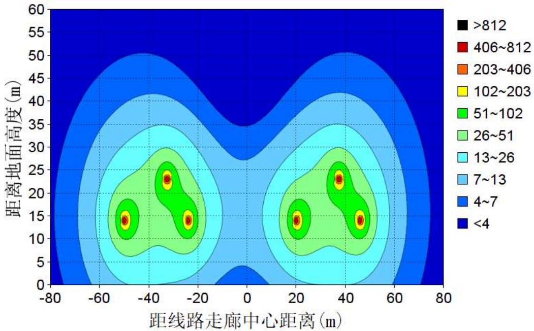
图 6-50 单回三角并行段对地高度 11m 的磁感应强度等值线图
