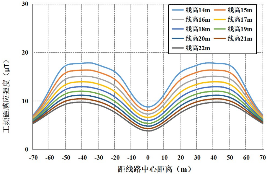
图 6-38 单回水平并行段在居民区最不利塔型磁感应强度随距离变化趋势图（离地 1.5m）
