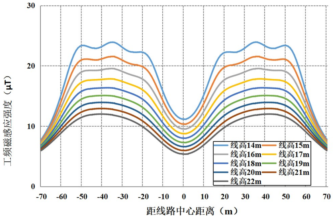
图 6-39 单回水平并行段在居民区最不利塔型磁感应强度随距离变化趋势图（离地 4.5m）
