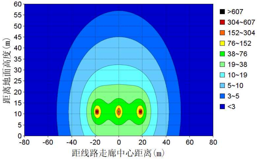
图 6-20 单回水平段对地高度 11m 的磁感应强度等值线图
