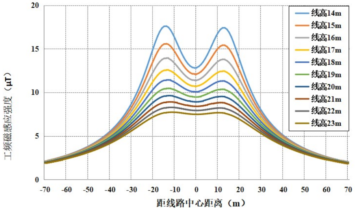
图 6-59 双回段线路在居民区最不利塔型磁感应强度随距离变化趋势图（离地 4.5m）
