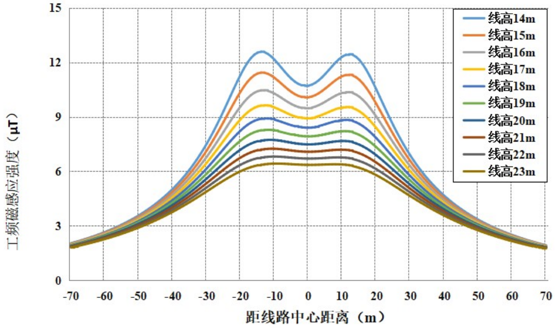
图 6-58 双回段线路在居民区最不利塔型磁感应强度随距离变化趋势图（离地 1.5m）
