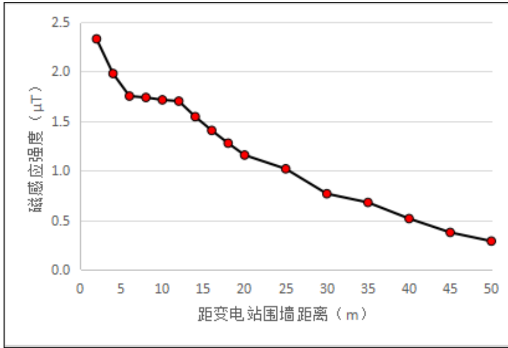
图 6-5 丹景 500kV 变电站围墙外磁感应强度随距离变化趋势图
