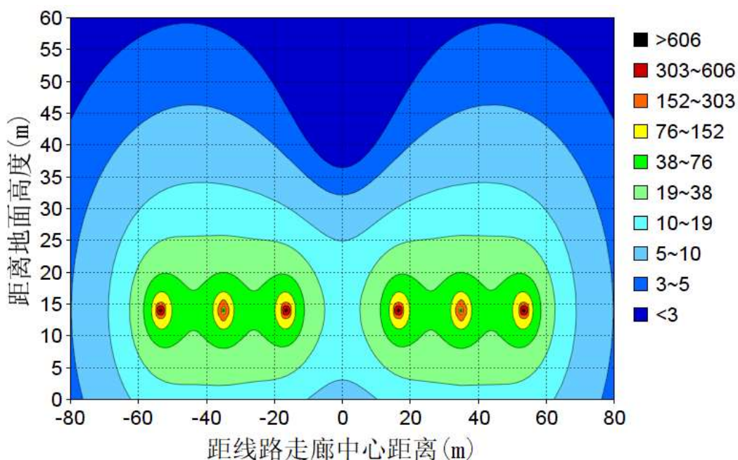
图 6-36 单回水平并行段对地高度 14m 的电场强度等值线图（单位：kV/m）
