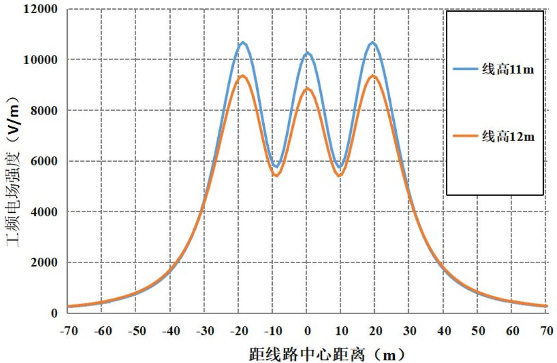
图 6-12 单回水平段线路通过非居民区最不利塔型电场强度随距离变化趋势图
