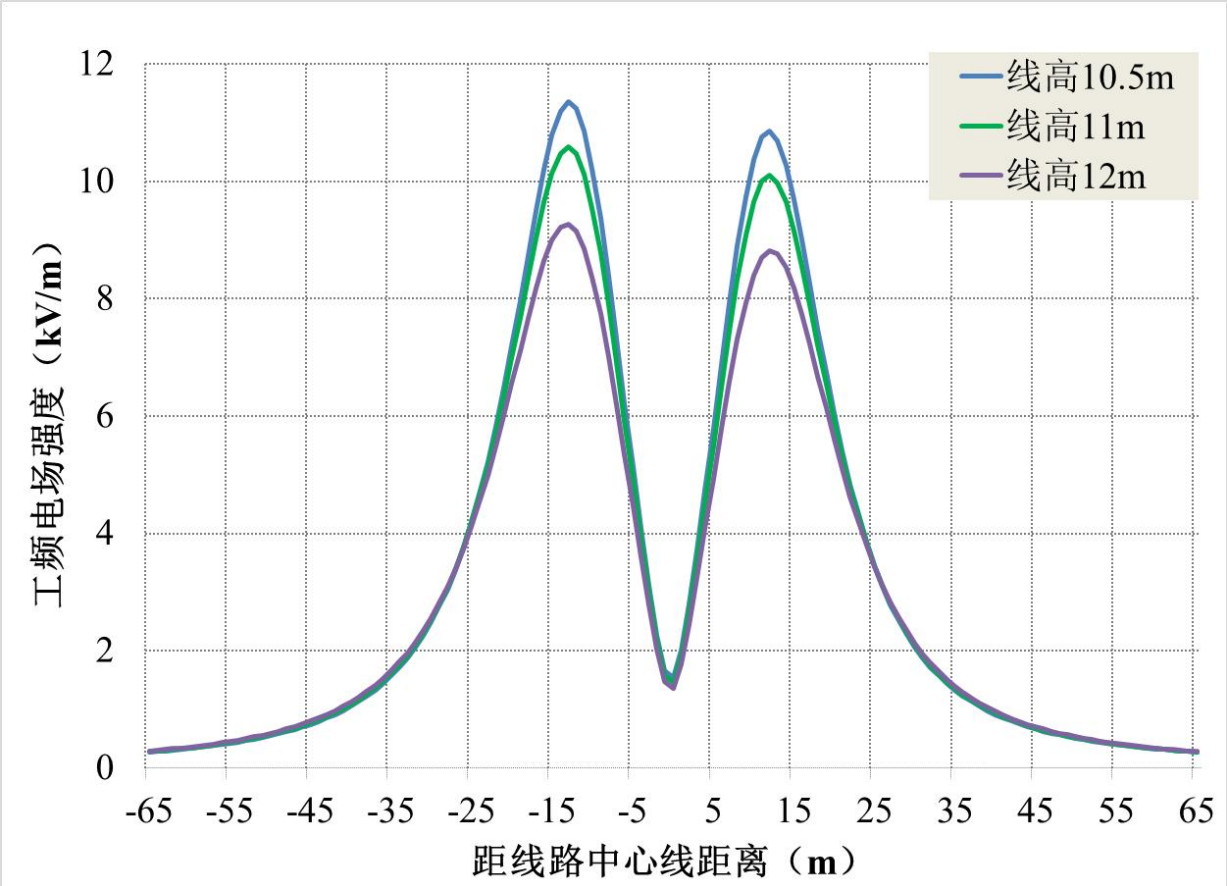
图 6-6 线路单回三角排列段通过耕地、园地、牧草地、畜禽饲养地、养殖水面、道路等场所最不利塔型电场强度随距离变化趋势图
