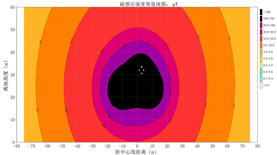
图 6.1-25 500kV 单回线路（三角排列）经过电磁环境敏感目标时工频磁感应强度达标等值线图
