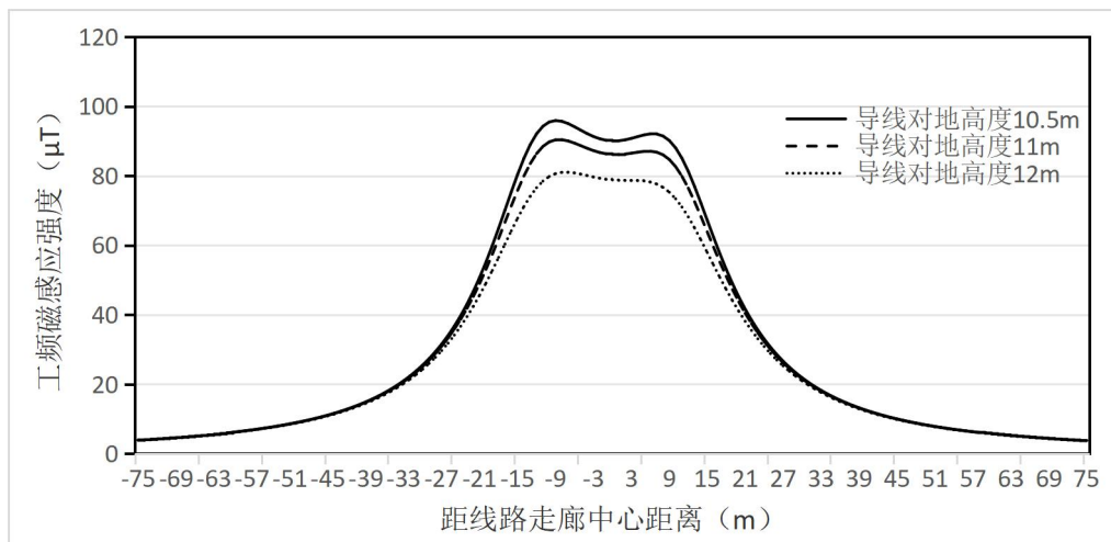
图 6.1-19 (2) 500kV 单回线路（三角排列）工频磁感应强度趋势线图
