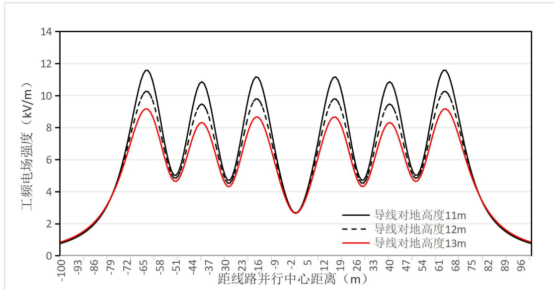
图 6.1-26 (1) 500kV 单回线路并行段工频电场强度趋势线
