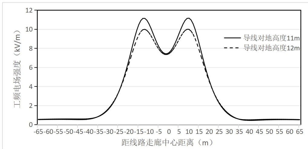
图 6.1-10 (1) 500kV 双回线路工频电场强度趋势线
