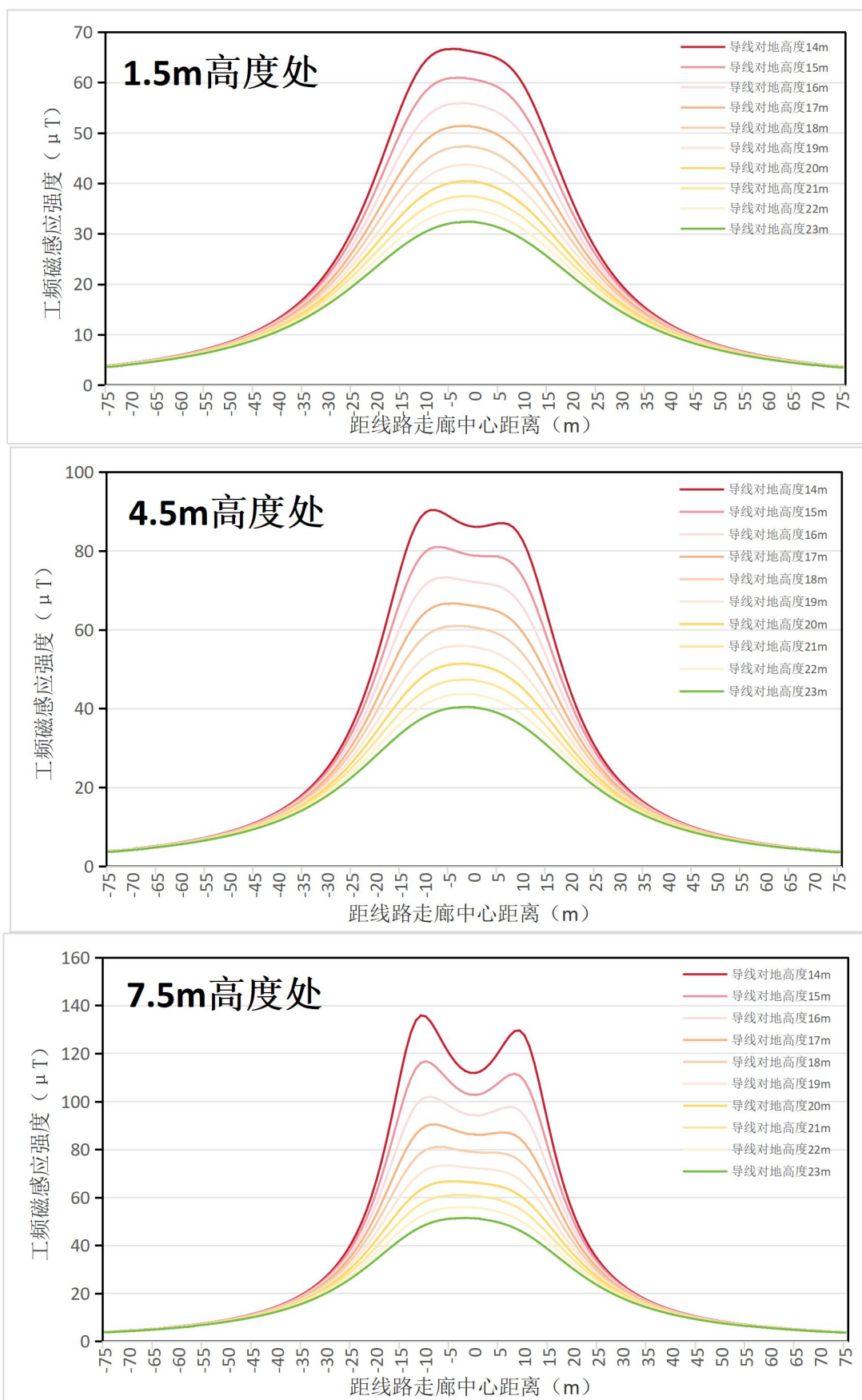
图 6.1-24 500kV 单回线路（三角排列）经过电磁环境敏感目标时工频磁感应强度趋势线图
