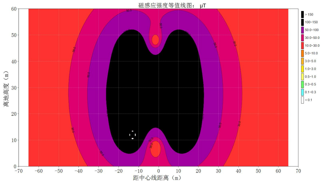
图 6.1-11 (2) 本期 500kV 双回线路工频磁感应强度达标等值线图
