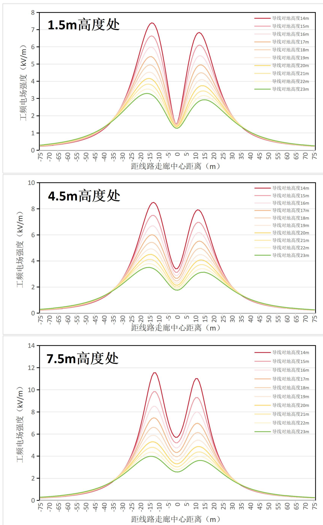
图 6.1-21 500kV 单回线路（三角排列）经过电磁环境敏感目标时工频电场强度趋势线图
