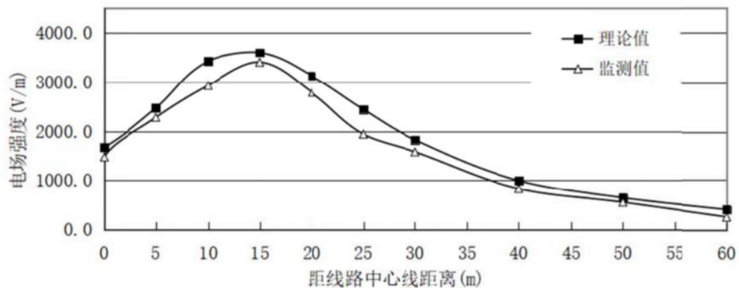
图 6.1-8 500kV 洪板二线工频电场强度监测值与预测值对比图
