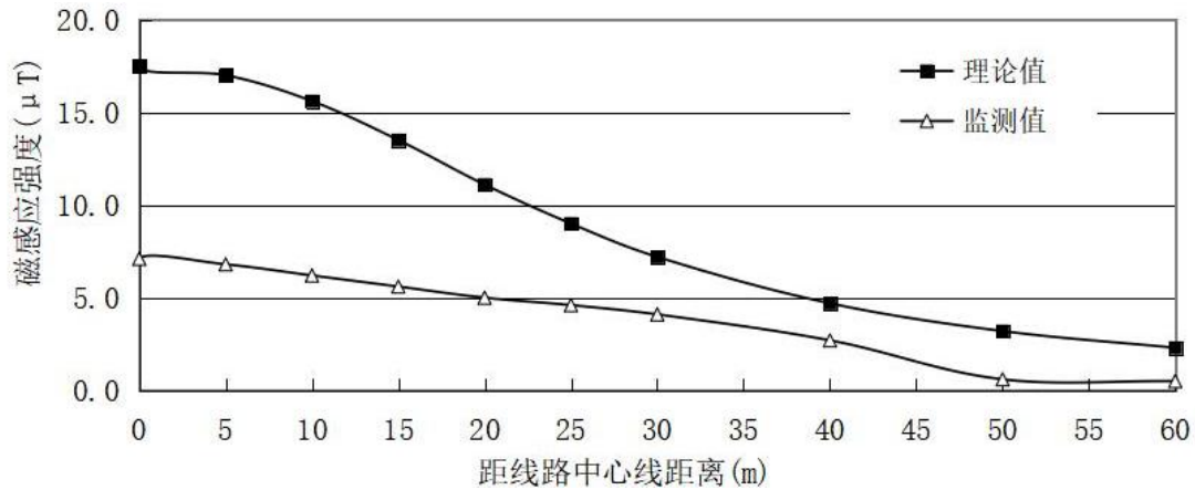
图 6.1-7 500kV 洪板一线工频磁感应强度监测值与预测值对比图
