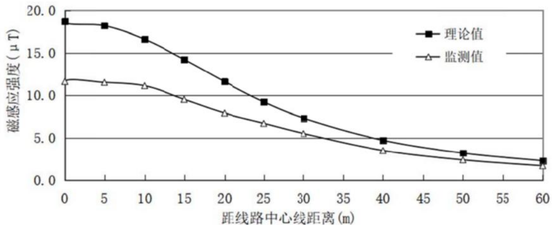
图 6.1-9 500kV 洪板二线工频磁感应强度监测值与预测值对比图
