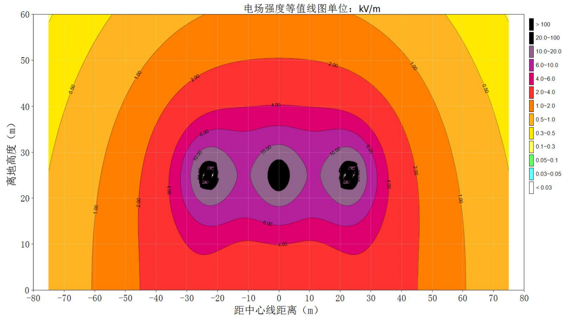
图 6.1-15 500kV 单回线路（水平排列）经过电磁环境敏感目标时工频电场强度达标等值线图
