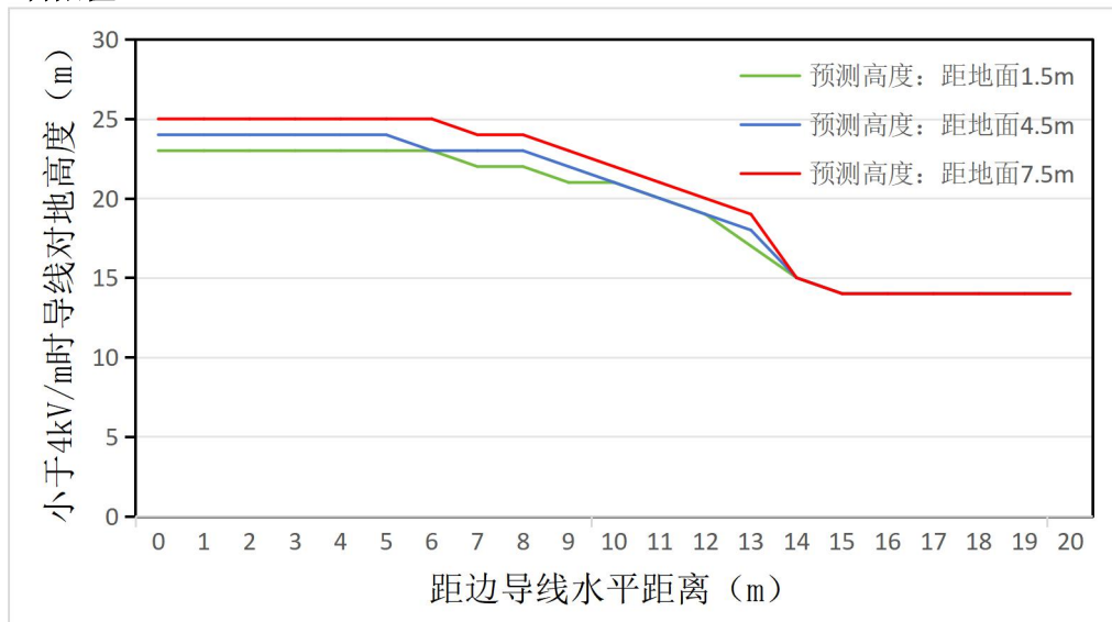
图 6.1-16 电磁环境敏感目标处距线路边导线不同距离相应最低导线高度关系图
