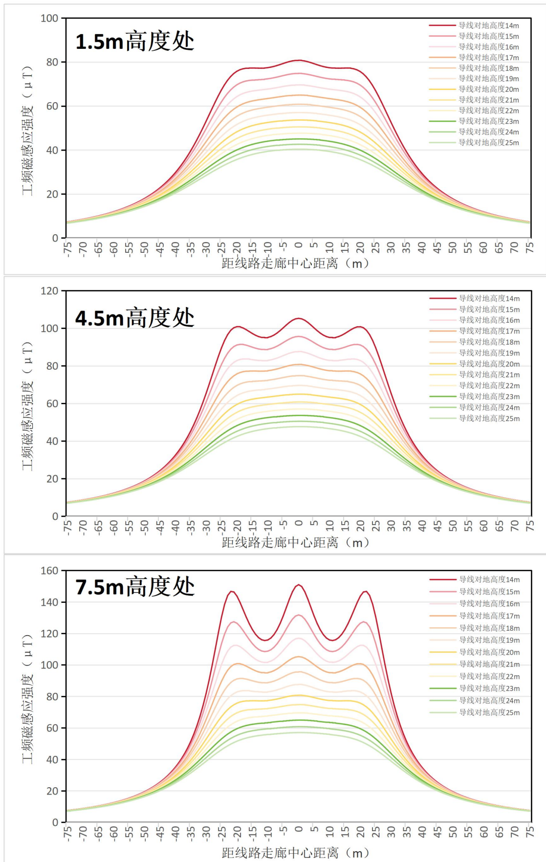
图 6.1-17 500kV 单回线路（水平排列）经过电磁环境敏感目标时工频磁感应强度趋势线图
