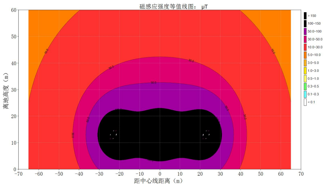
图 6.1-13 (2) 本期 500kV 单回线路（水平排列）工频磁感应强度达标等值线图
