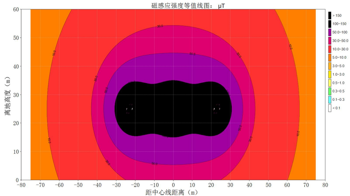
图 6.1-18 500kV 单回线路（水平排列）经过电磁环境敏感目标时工频磁感应强度达标等值线图
