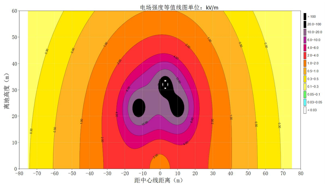
图 6.1-22 500kV 单回线路（三角排列）经过电磁环境敏感目标时工频电场强度达标等值线图
