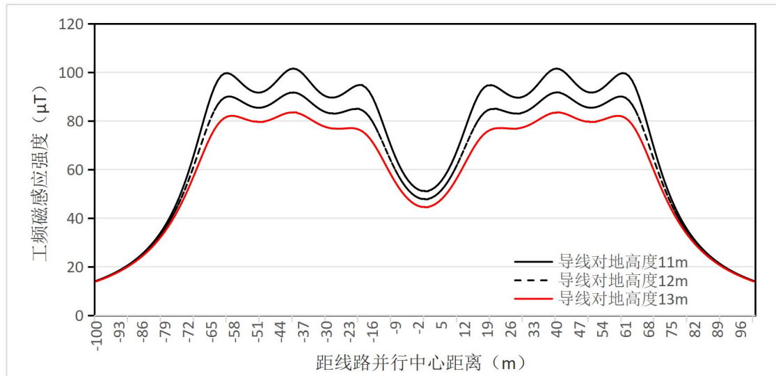
图 6.1-26 (2) 500kV 单回线路并行段工频磁感应强度趋势线
