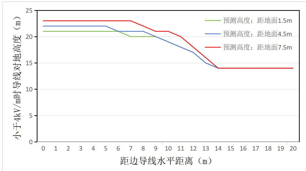
图 6.1-23 电磁环境敏感目标处距线路边导线不同距离相应最低导线高度关系图
