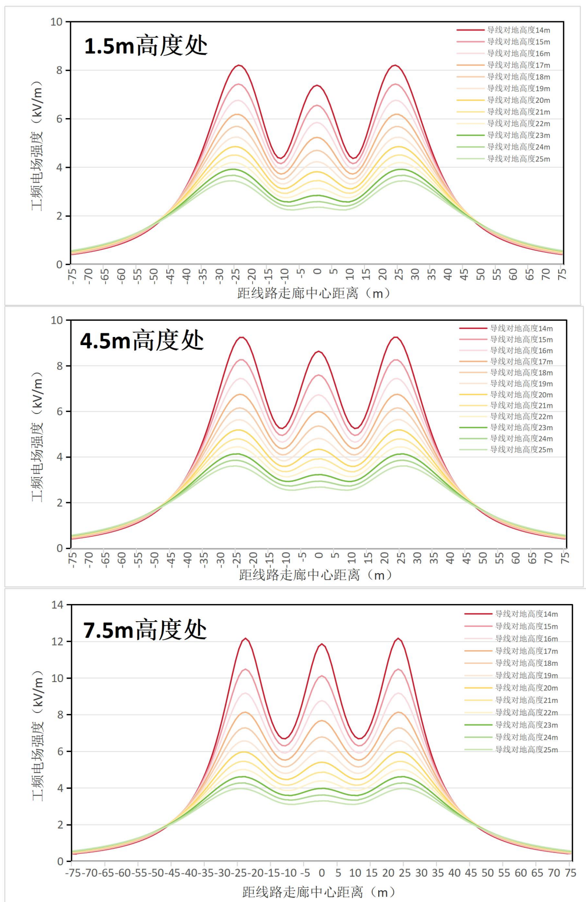
图 6.1-14 500kV 单回线路（水平排列）经过电磁环境敏感目标时工频电场强度趋势线图
