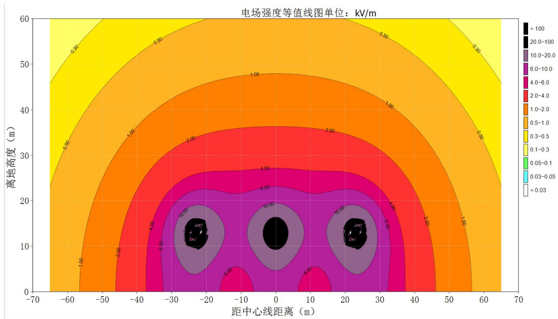
图 6.1-13 (1) 本期 500kV 单回线路（水平排列）工频电场强度达标等值线图
