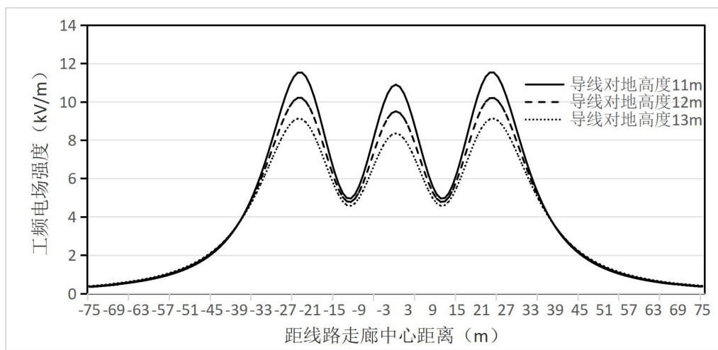
图 6.1-12 (1) 500kV 单回线路（水平排列）工频电场强度趋势线图
