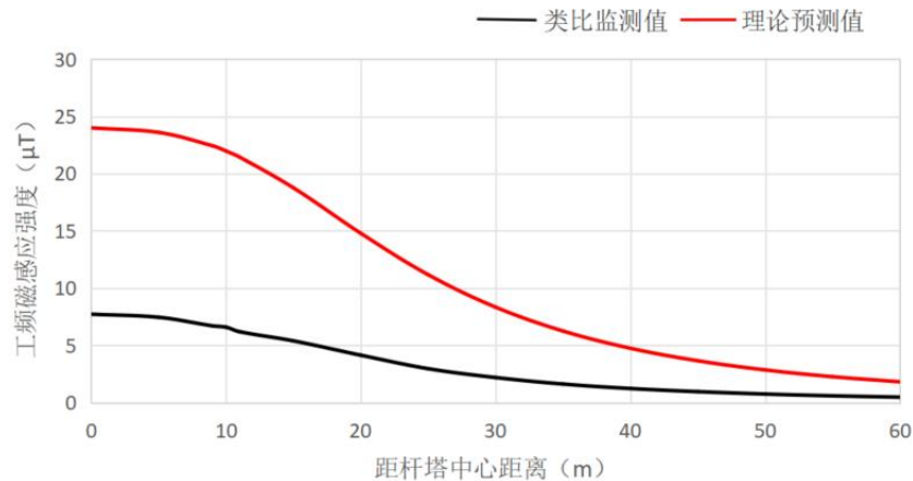
图 6.1-5 500kV 茂谭一线/二线工频磁感应强度监测值与预测值对比图
