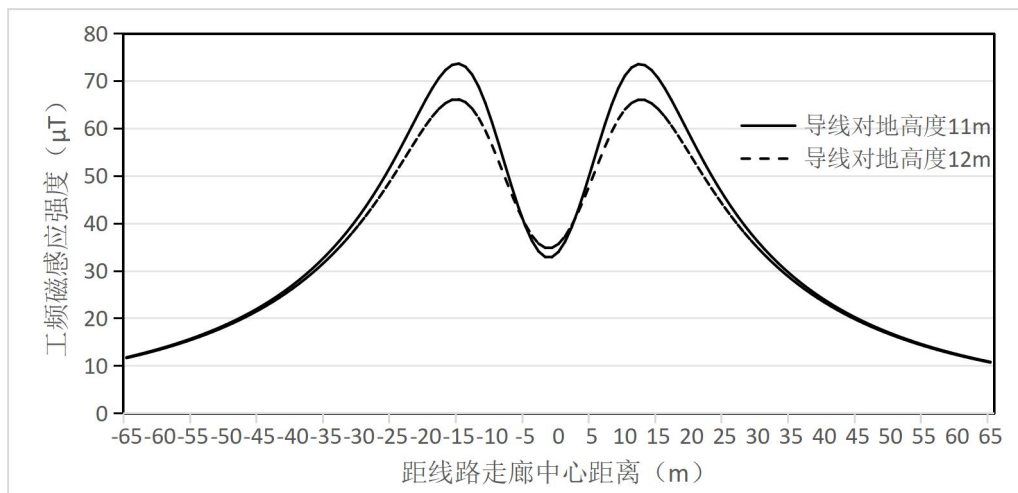
图 6.1-10 (2) 500kV 双回线路工频磁感应强度趋势线
