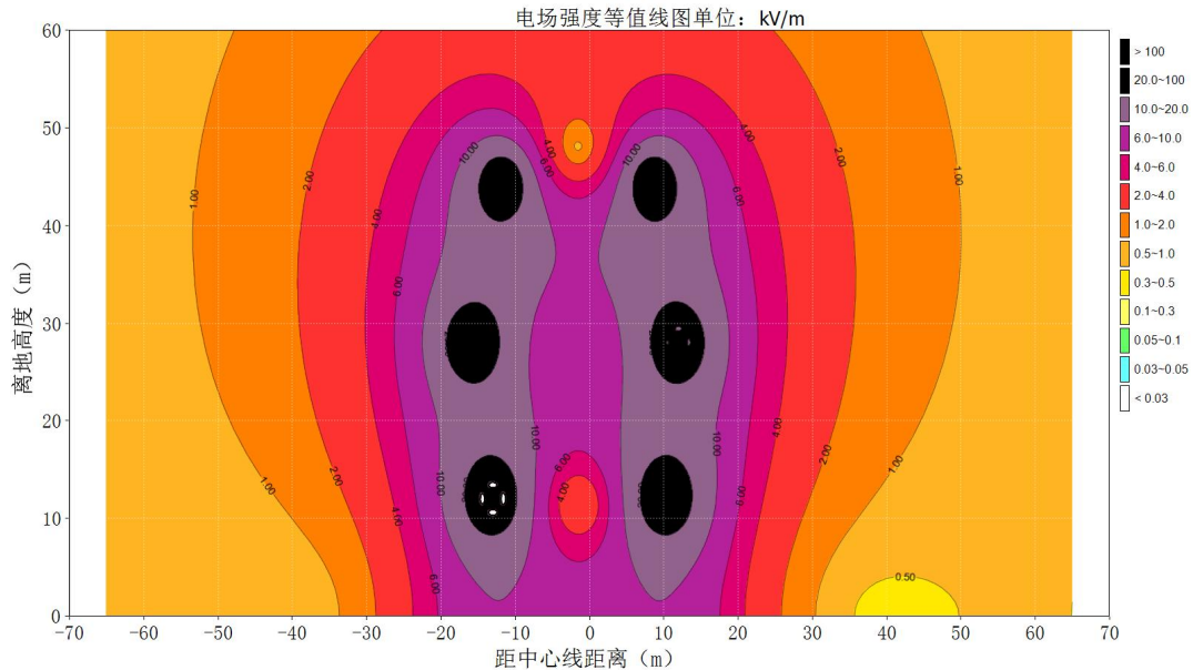
图 6.1-11 (1) 本期 500kV 双回线路工频电场强度达标等值线图
