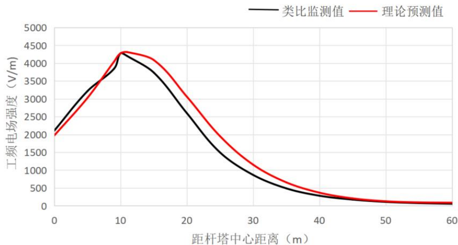
图 6.1-4 500kV 茂谭一线/二线工频电场强度监测值与预测值对比图
