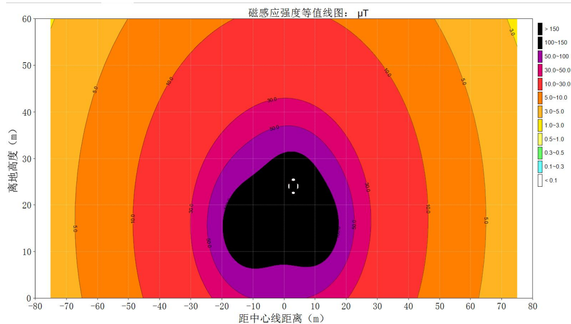
图 6.1-20 (2) 本期 500kV 单回线路（三角排列）工频磁感应强度达标等值线图
