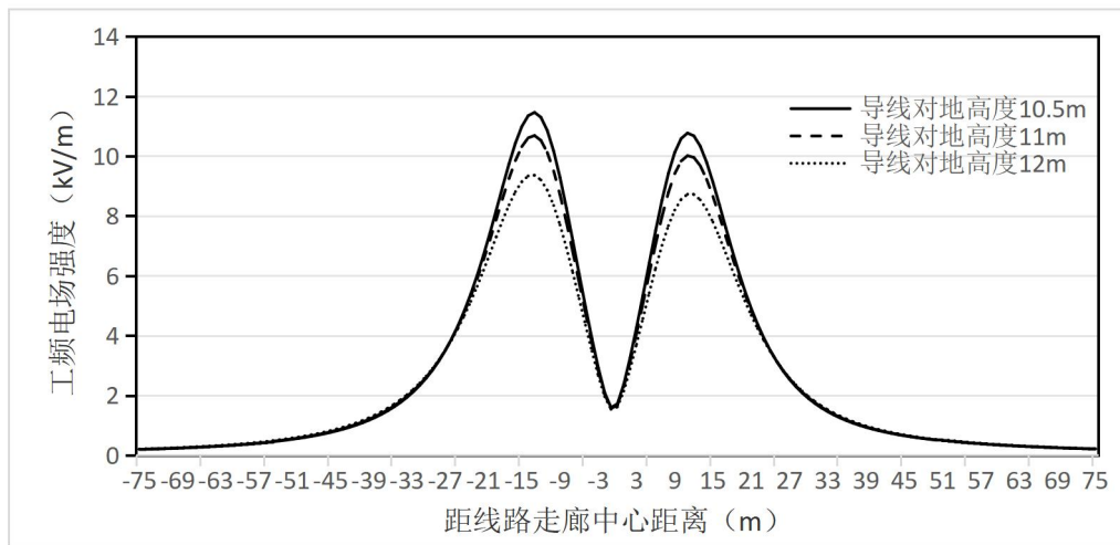
图 6.1-19 (1) 500kV 单回线路（三角排列）工频电场强度趋势线图
