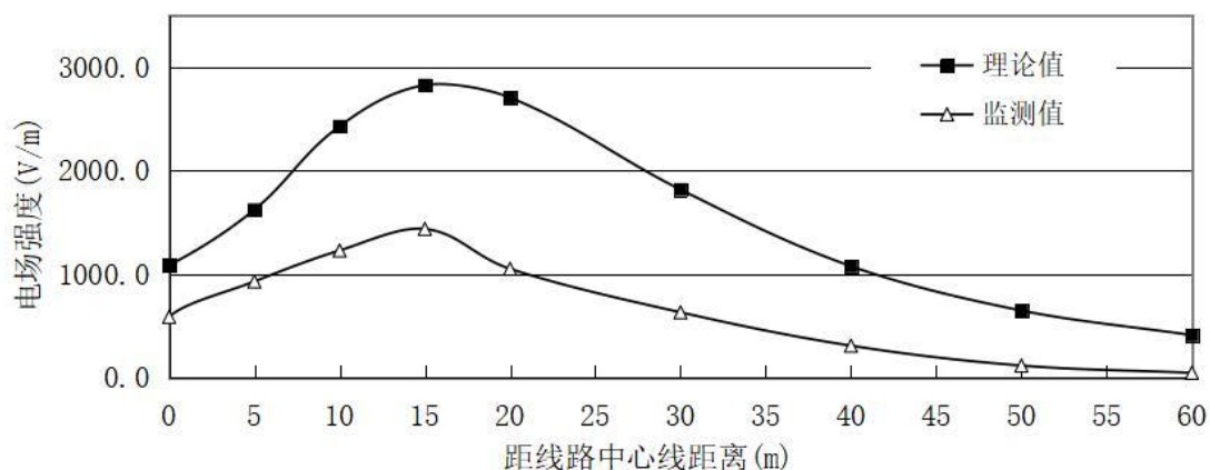
图 6.1-6 500kV 洪板一线工频电场强度监测值与预测值对比图
