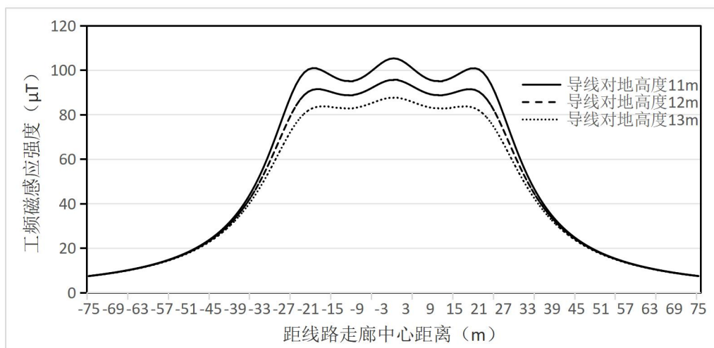
图 6.1-12 (2) 500kV 单回线路（水平排列）工频磁感应强度趋势线图
