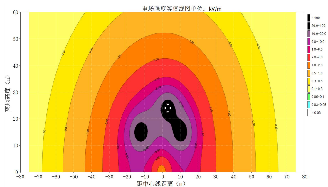
图 6.1-20 (1) 本期 500kV 单回线路（三角排列）工频电场强度达标等值线图
