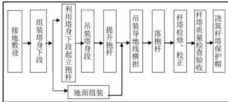
图 3.1-3 杆塔组立施工流程图
