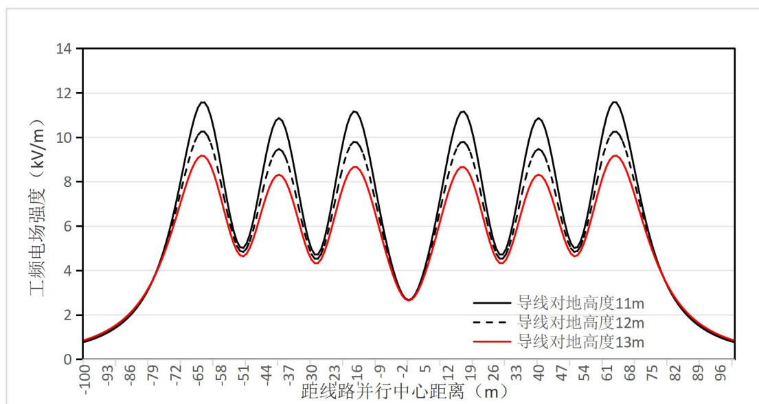
图 6.1-29 (1) 两条水平排列 500kV 单回线路并行段工频电场强度趋势线
