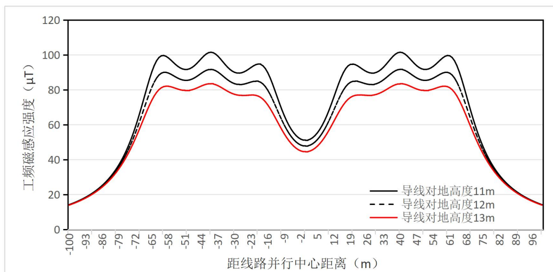
图 6.1-29 (2) 两条水平排列 500kV 单回线路并行段工频磁感应强度趋势线
