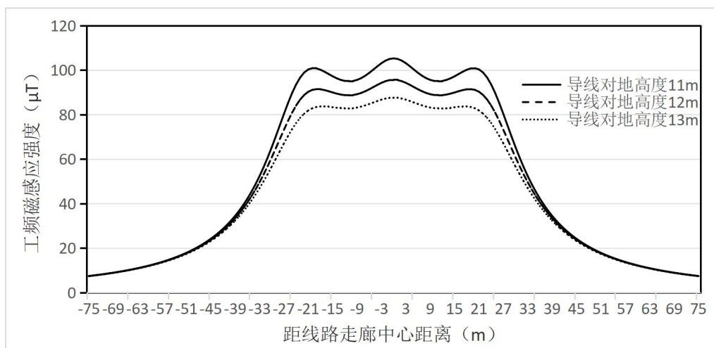
图 6.1-15 (2) 500kV 单回线路（水平排列）工频磁感应强度趋势线图
