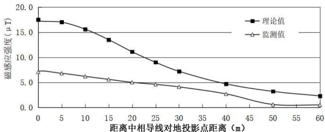
图 6.1-10 500kV 洪板一线工频磁感应强度监测值与预测值对比图
