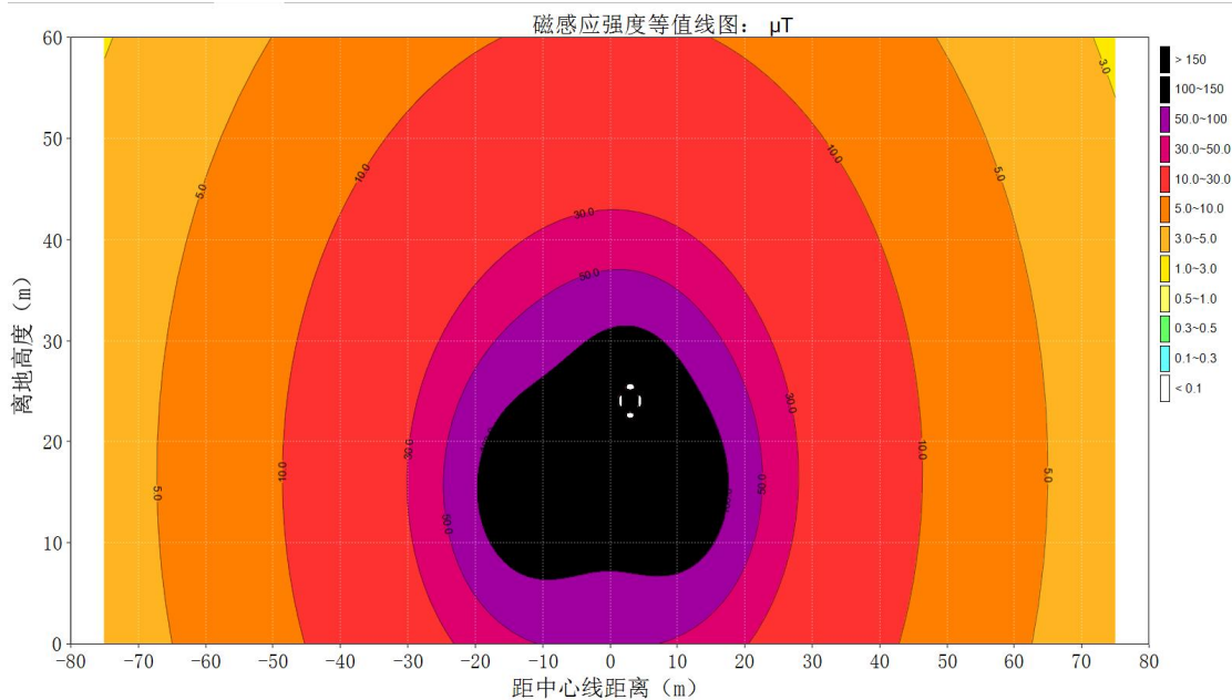
图 6.1-23 (2) 本期 500kV 单回线路（三角排列）工频磁感应强度达标等值线图
