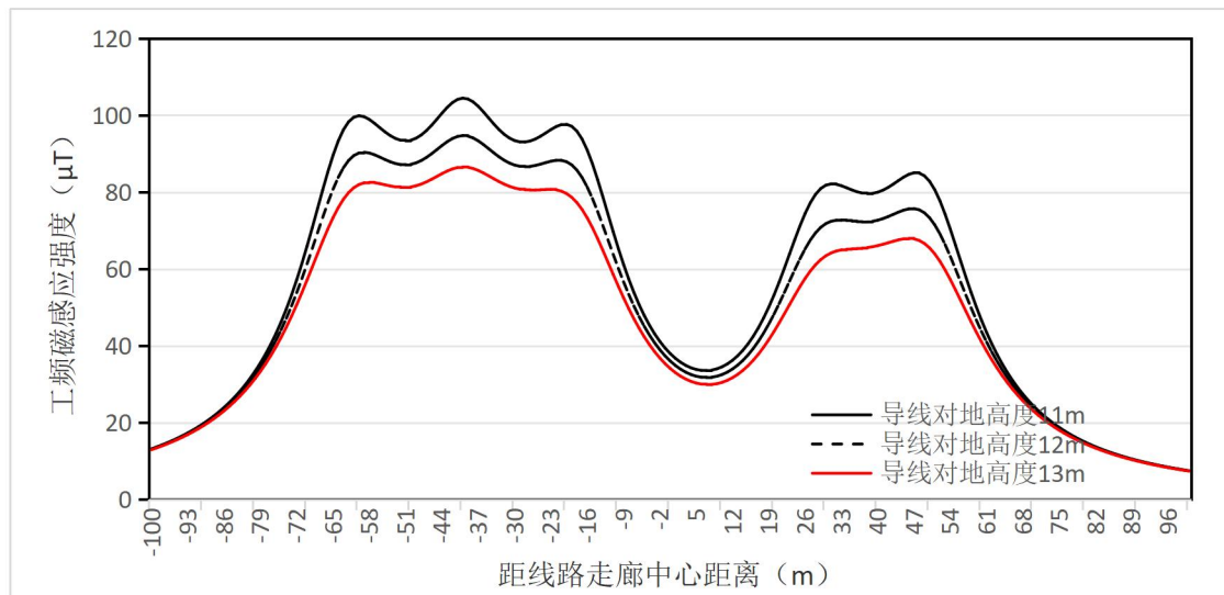
图 6.1-33 (2) 500kV 水平排列与三角排列单回线路并行段工频磁感应强度趋势线
