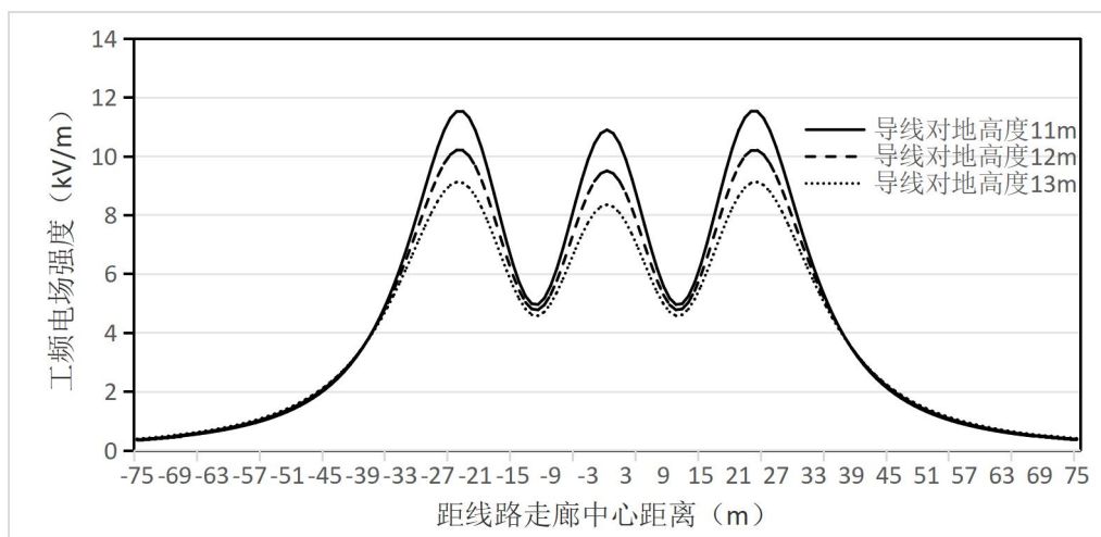
图 6.1-15 (1) 500kV 单回线路（水平排列）工频电场强度趋势线图
