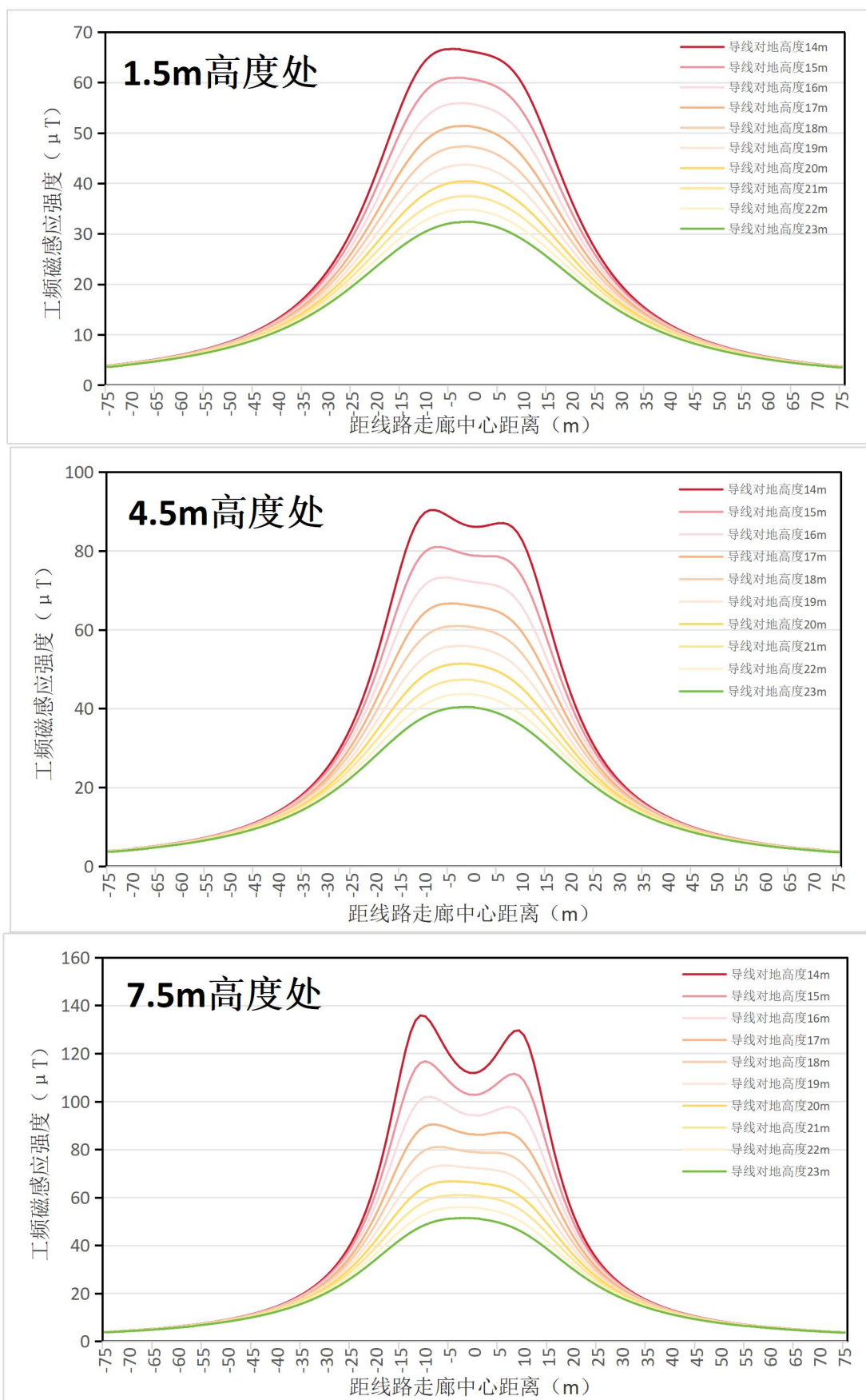
图 6.1-27 500kV 单回线路（三角排列）经过电磁环境敏感目标时工频磁感应强度趋势线图
