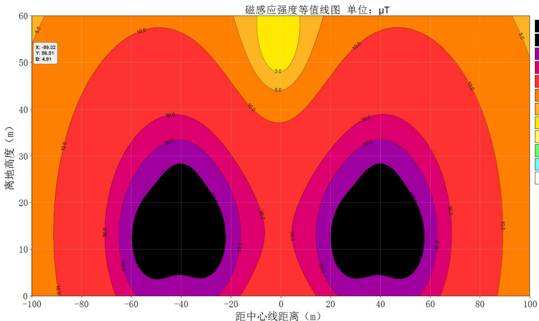
图 6.1-32 (2) 两条三角排列 500kV 单回线路并行段工频磁感应强度等值线图
