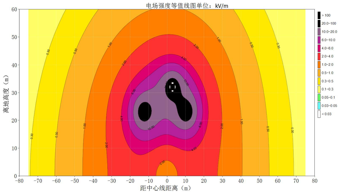
图 6.1-25 500kV 单回线路（三角排列）经过电磁环境敏感目标时工频电场强度达标等值线图
