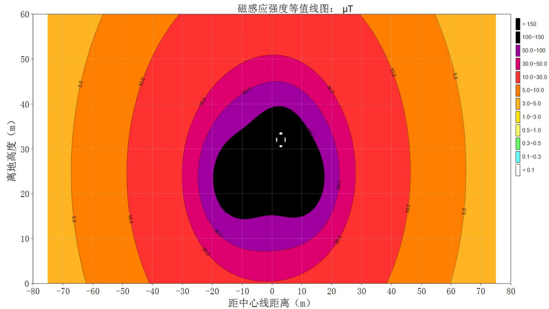
图 6.1-28 500kV 单回线路（三角排列）经过电磁环境敏感目标时工频磁感应强度达标等值线图
