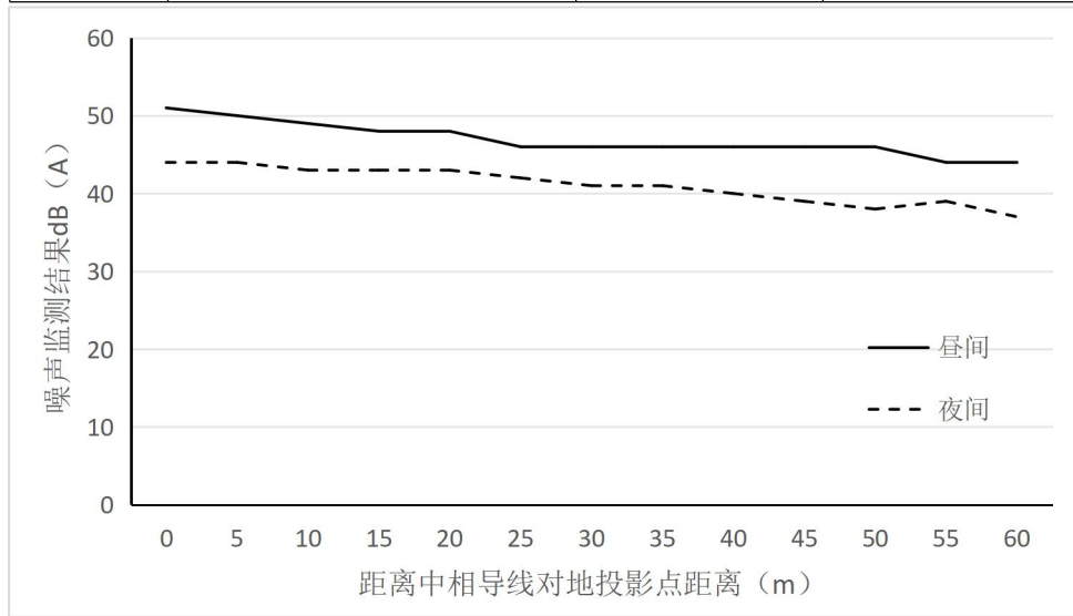
图 6.2-3 500kV 洪板二线噪声度随距中心线距离变化趋势图
