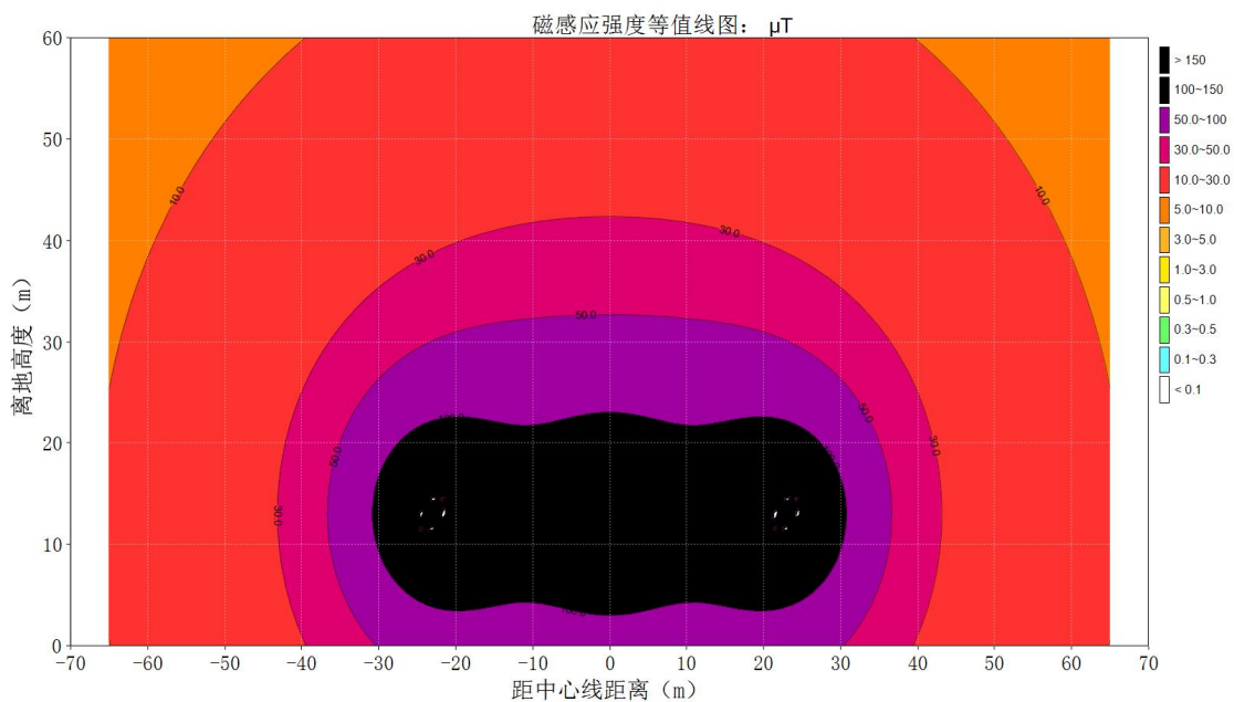
图 6.1-16 (2) 本期 500kV 单回线路（水平排列）工频磁感应强度达标等值线图
