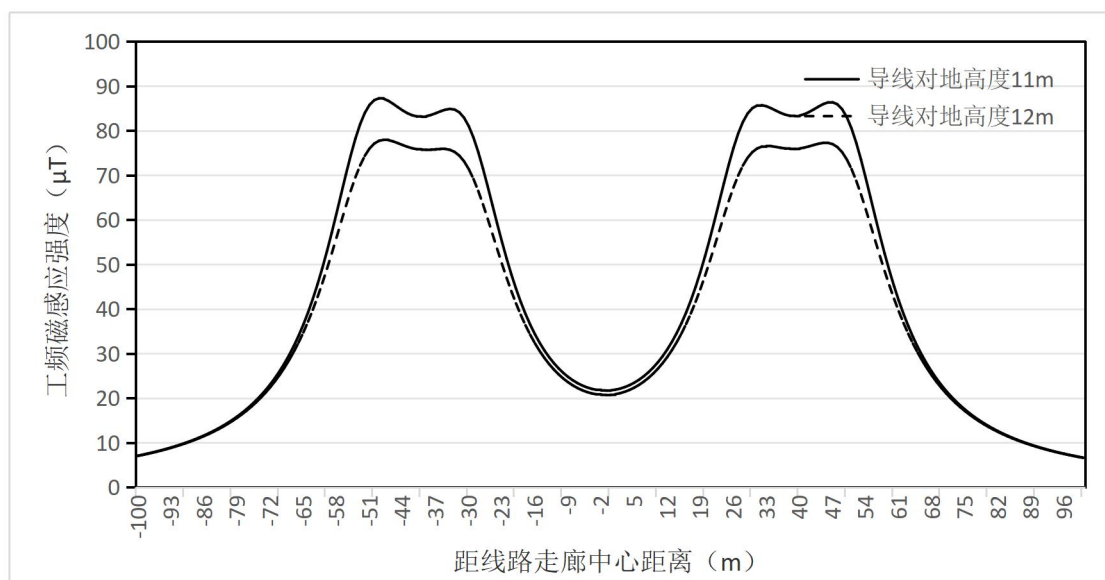
图 6.1-31 (2) 两条三角排列 500kV 单回线路并行段工频磁感应强度趋势线
