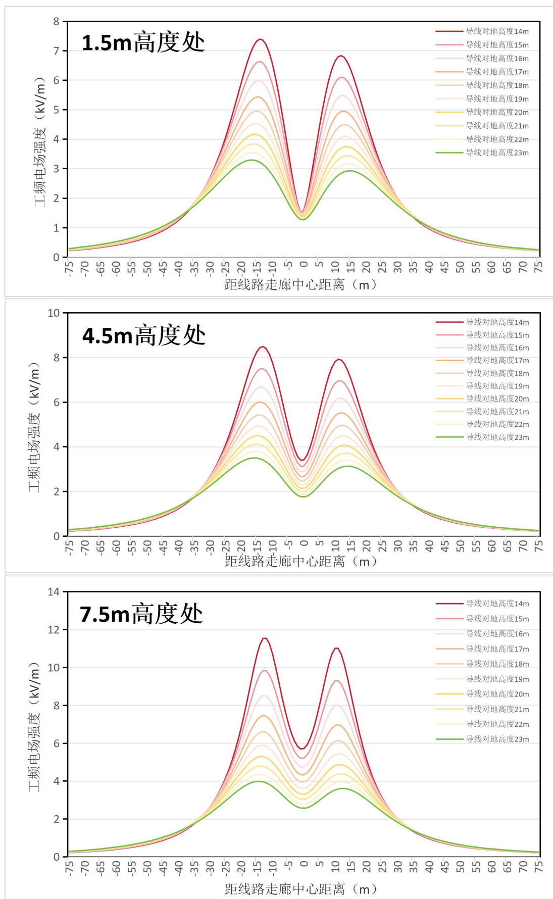
图 6.1-24 500kV 单回线路（三角排列）经过电磁环境敏感目标时工频电场强度趋势线图
