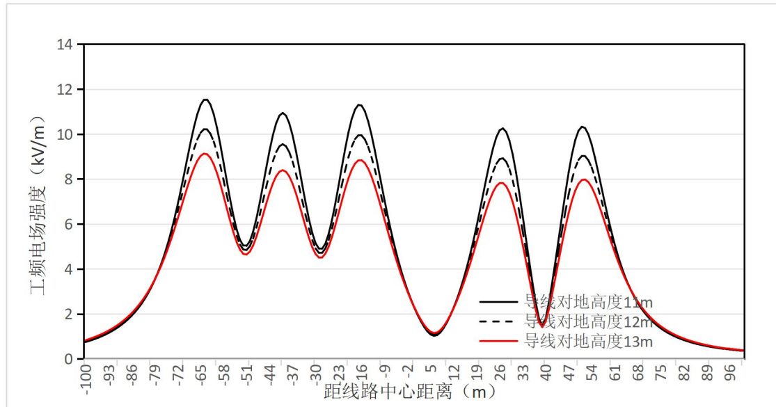
图 6.1-33 (1) 500kV 水平排列与三角排列单回线路并行段工频电场强度趋势线
