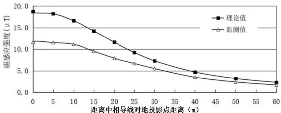
图 6.1-12 500kV 洪板二线工频磁感应强度监测值与预测值对比图
