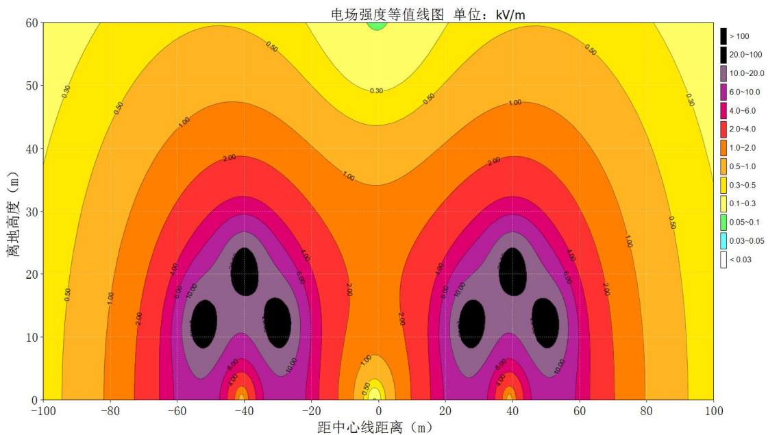
图 6.1-32 (1) 两条三角排列 500kV 单回线路并行段工频电场强度达标等值线图
