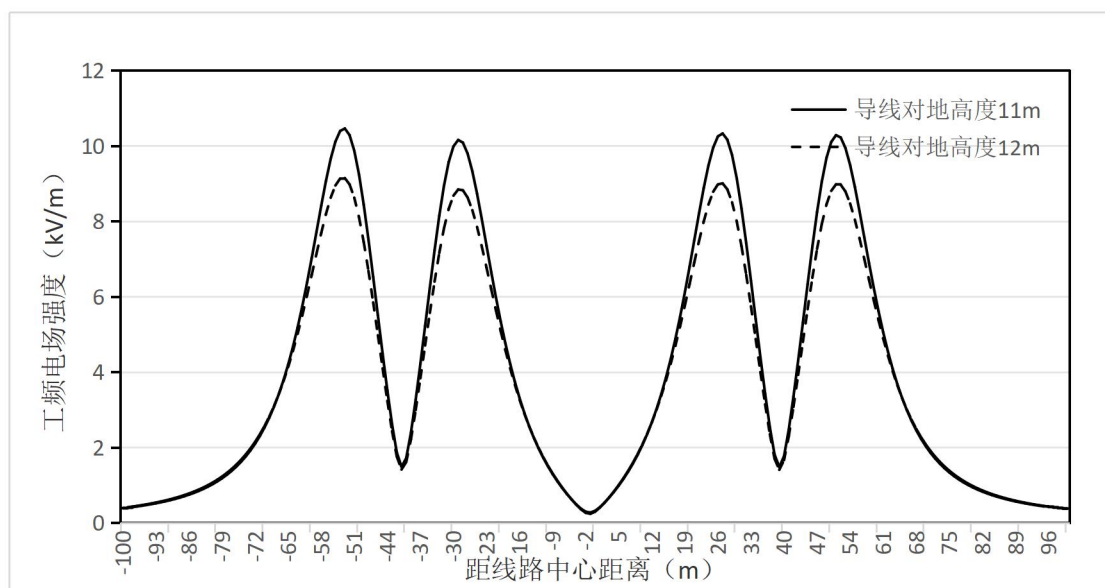
图 6.1-31 (1) 两条三角排列 500kV 单回线路并行段工频电场强度趋势线
