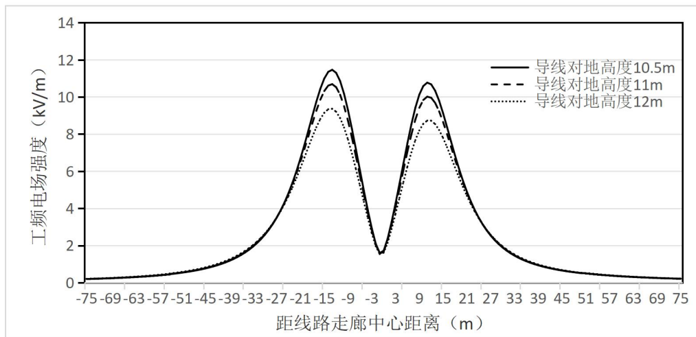
图 6.1-22 (1) 500kV 单回线路（三角排列）工频电场强度趋势线图
