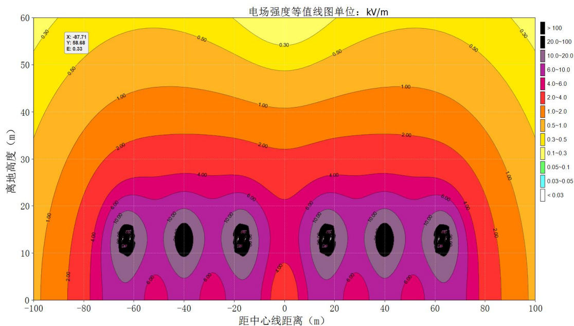
图 6.1-30 (1) 两条水平排列 500kV 单回线路并行段工频电场强度达标等值线图
