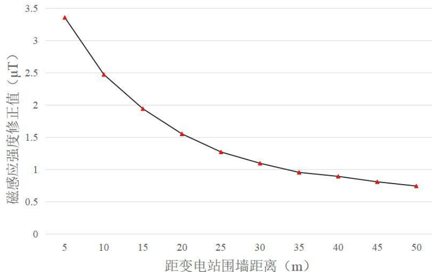
图 6.1-3 广都 500kV 变电站南侧断面工频磁感应强度变化趋势示意图
