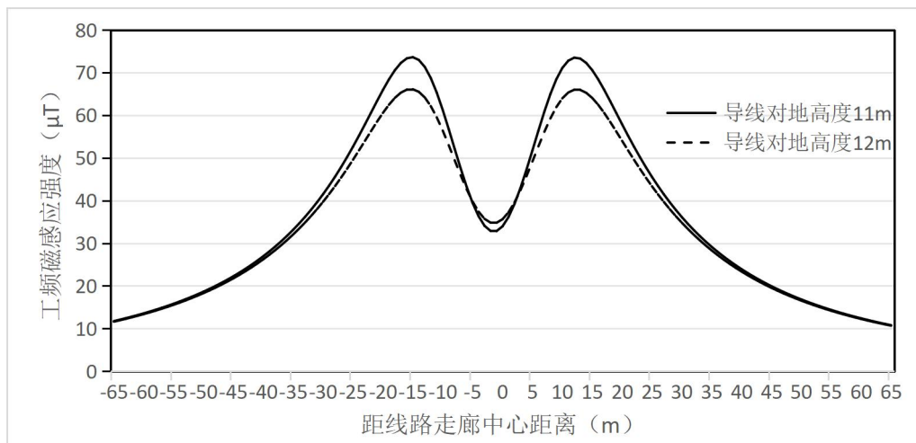
图 6.1-13 (2) 500kV 双回线路工频磁感应强度趋势线
