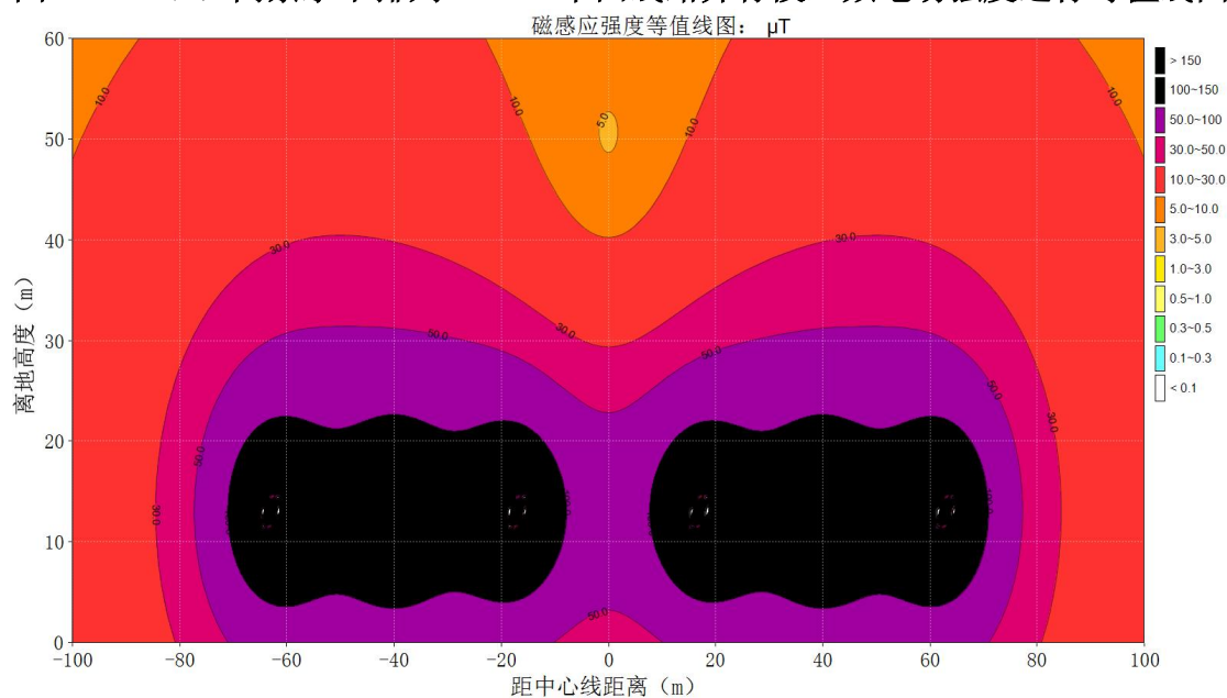
图 6.1-30 (2) 两条水平排列 500kV 单回线路并行段工频磁感应强度等值线图
