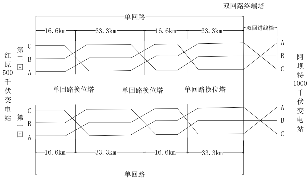
图 3.1-2 本项目输电线路相序一览图
