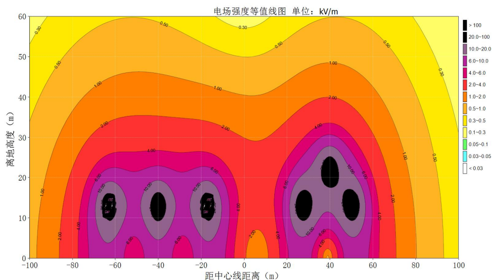
图 6.1-34 (1) 本期 500kV 水平排列与三角排列单回线路并行段工频电场强度达标等值线图
