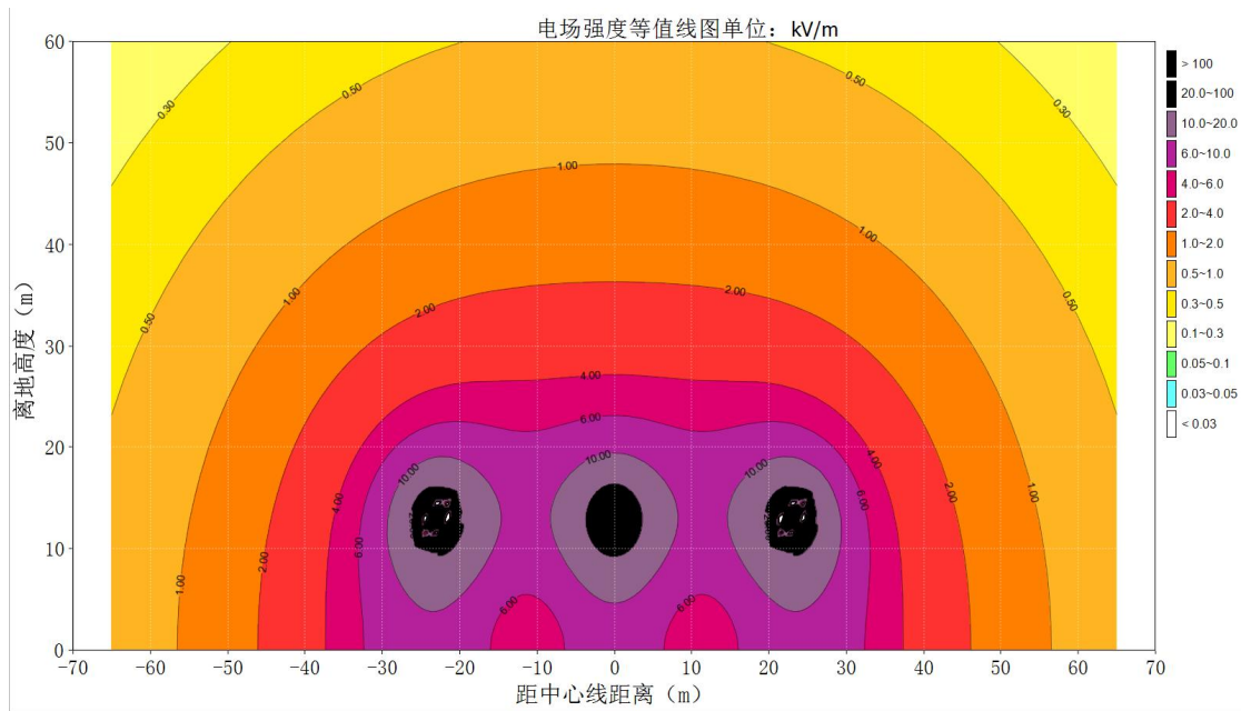
图 6.1-16 (1) 本期 500kV 单回线路（水平排列）工频电场强度达标等值线图
