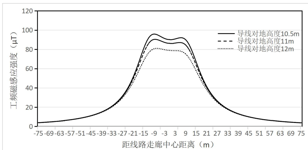
图 6.1-22 (2) 500kV 单回线路（三角排列）工频磁感应强度趋势线图
