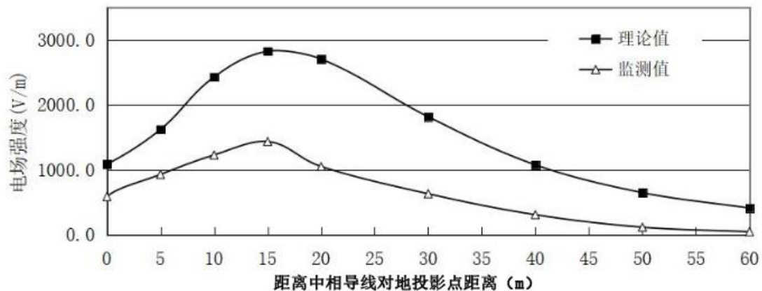
图 6.1-9 500kV 洪板一线工频电场强度监测值与预测值对比图
