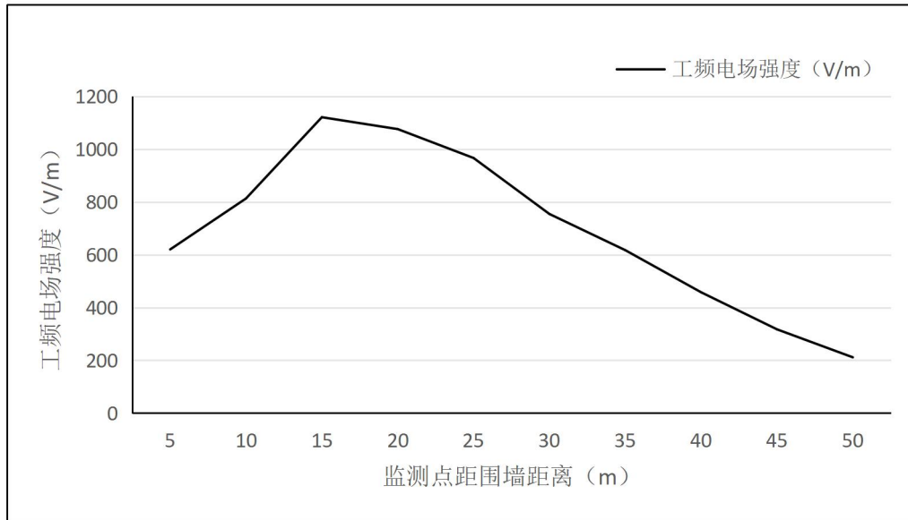
图 6.1-5 济南 1000kV 变电站衰减断面工频电场强度变化趋势示意图
