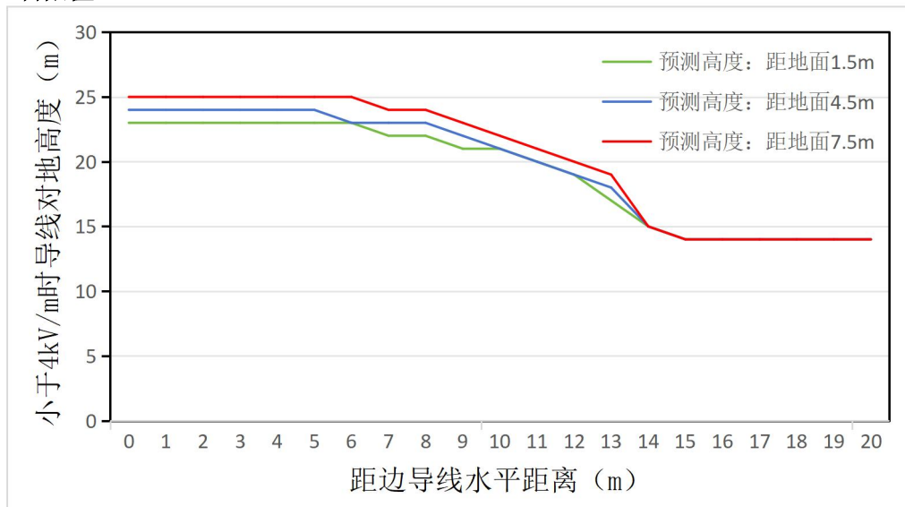
图 6.1-19 电磁环境敏感目标处距线路边导线不同距离相应最低导线高度关系图
