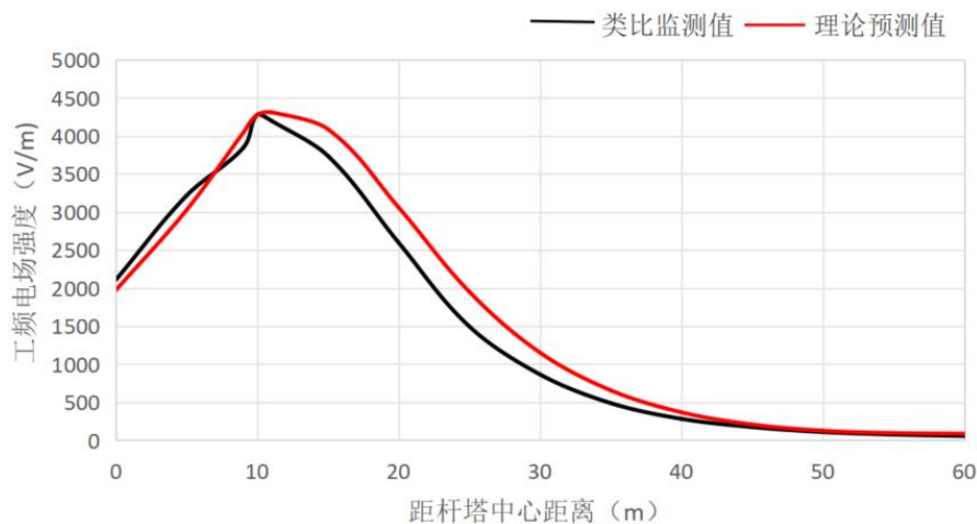
图 6.1-7 500kV 茂谭一线/二线工频电场强度监测值与预测值对比图
