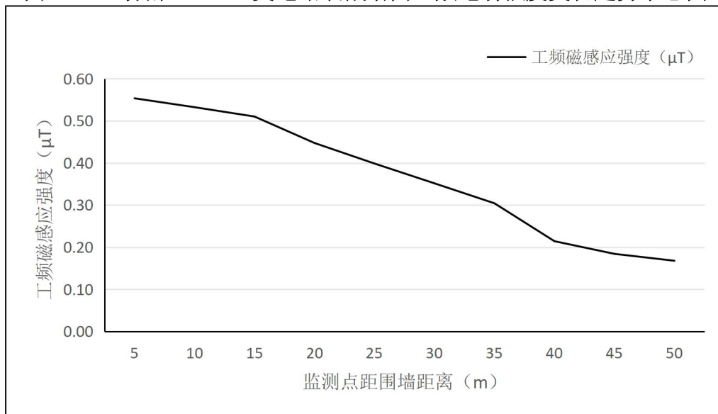
图 6.1-6 济南 1000kV 变电站衰减断面工频磁感应强度变化趋势示意图
