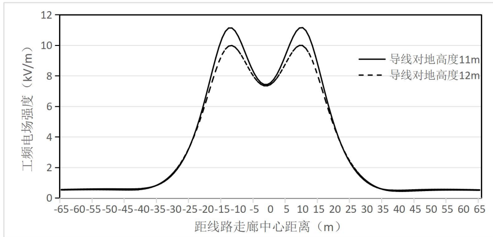
图 6.1-13 (1) 500kV 双回线路工频电场强度趋势线
