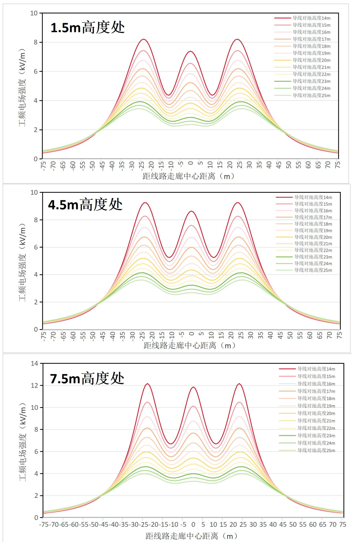
图 6.1-17 500kV 单回线路（水平排列）经过电磁环境敏感目标时工频电场强度趋势线图
