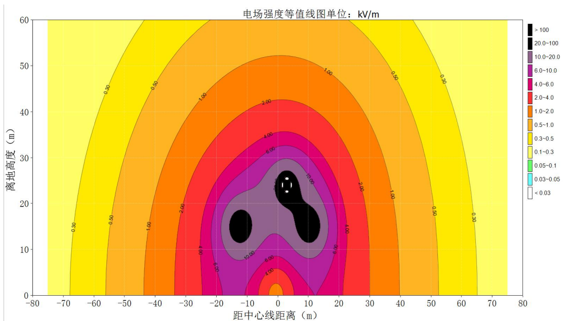
图 6.1-23 (1) 本期 500kV 单回线路（三角排列）工频电场强度达标等值线图
