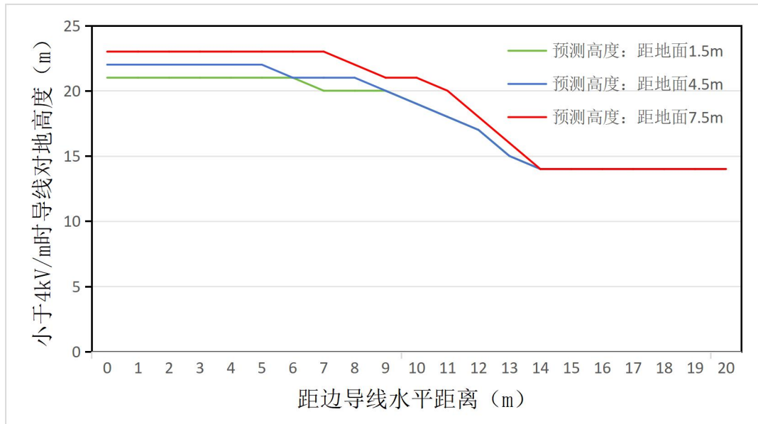
图 6.1-26 电磁环境敏感目标处距线路边导线不同距离相应最低导线高度关系图
