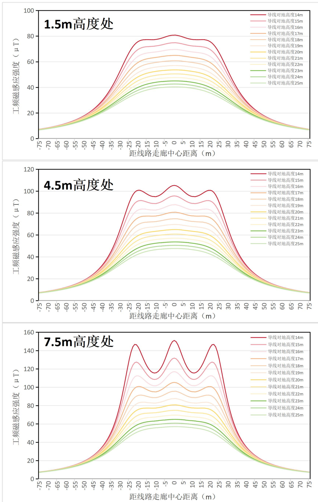
图 6.1-20 500kV 单回线路（水平排列）经过电磁环境敏感目标时工频磁感应强度趋势线图
