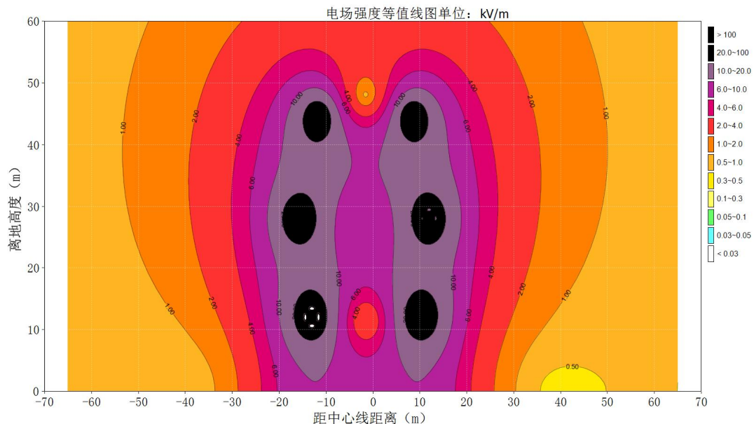
图 6.1-14 (1) 本期 500kV 双回线路工频电场强度达标等值线图
