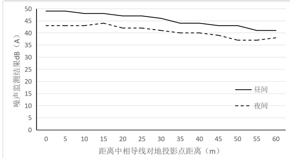
图 6.2-4 500kV 洪板一线噪声度随距中心线距离变化趋势图
