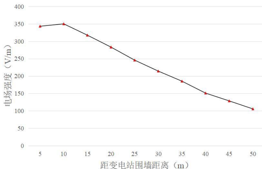
图 6.1-2 广都 500kV 变电站南侧断面工频电场强度变化趋势示意图
