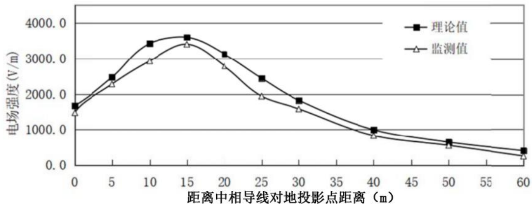
图 6.1-11 500kV 洪板二线工频电场强度监测值与预测值对比图
