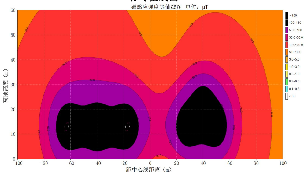
图 6.1-34 (2) 本期 500kV 水平排列与三角排列单回线路并行段工频磁感应强度达标等值线图
