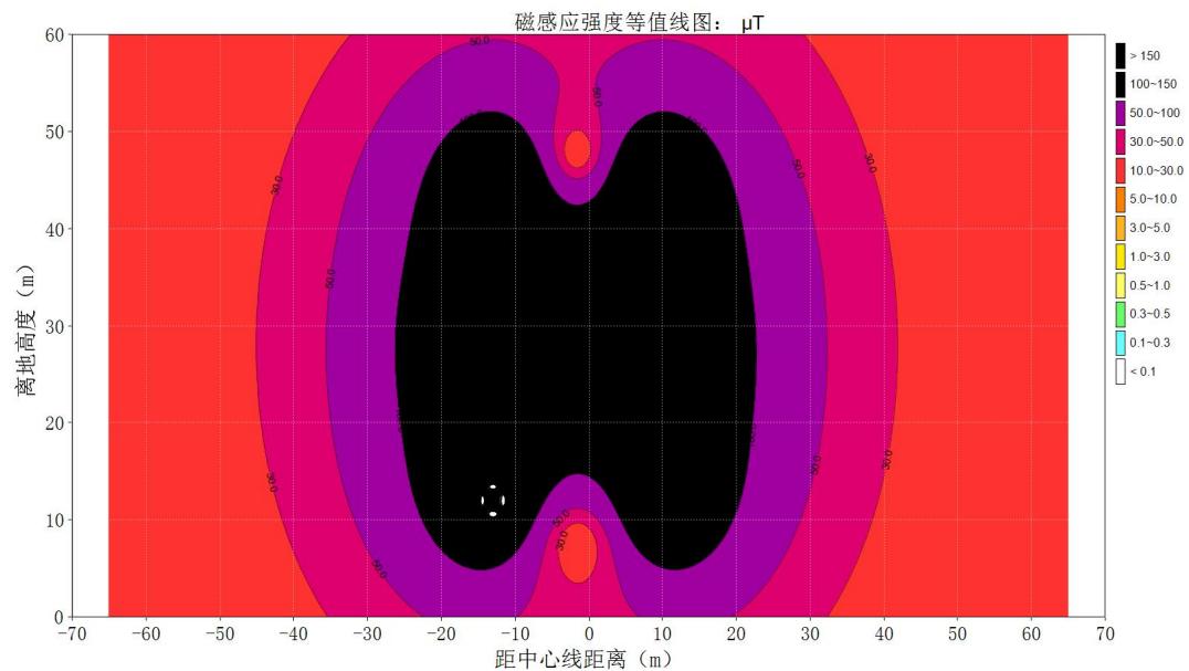
图 6.1-14 (2) 本期 500kV 双回线路工频磁感应强度达标等值线图
