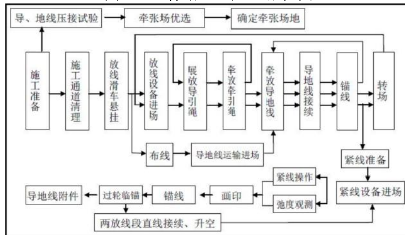
图 3.1-4 架线施工流程图
