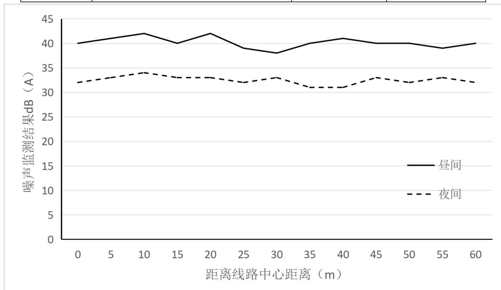
图 6.2-2 500kV 茂谭一线/茂谭二线噪声度随距中心线距离变化趋势图
