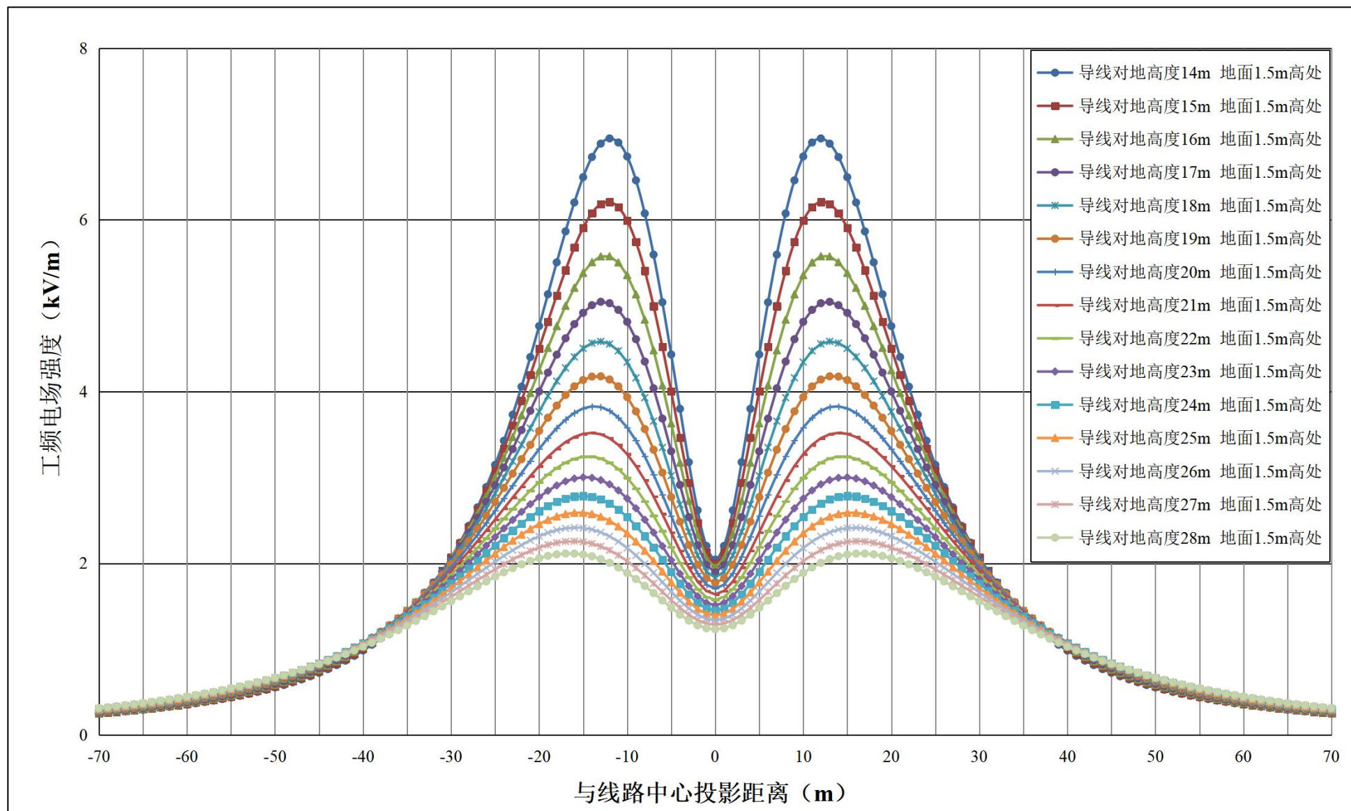
图 6.1-5 新建单回线路经过居民区时工频电场强度随距离变化趋势图（距地面 1.5m 高处）
