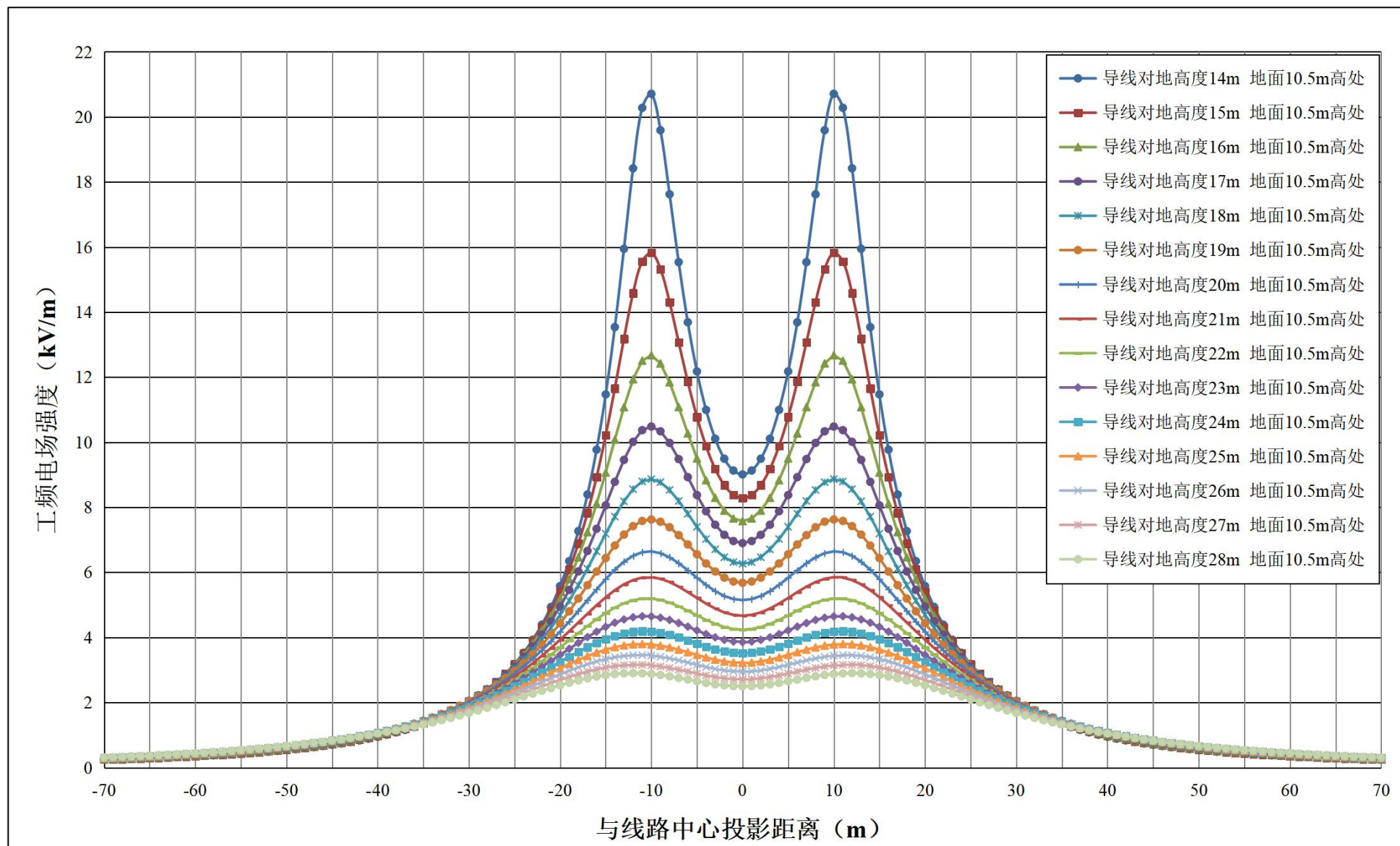
图 6.1-8 新建单回线路经过居民区时工频电场强度随距离变化趋势图 (距地面 10.5m 高处)
