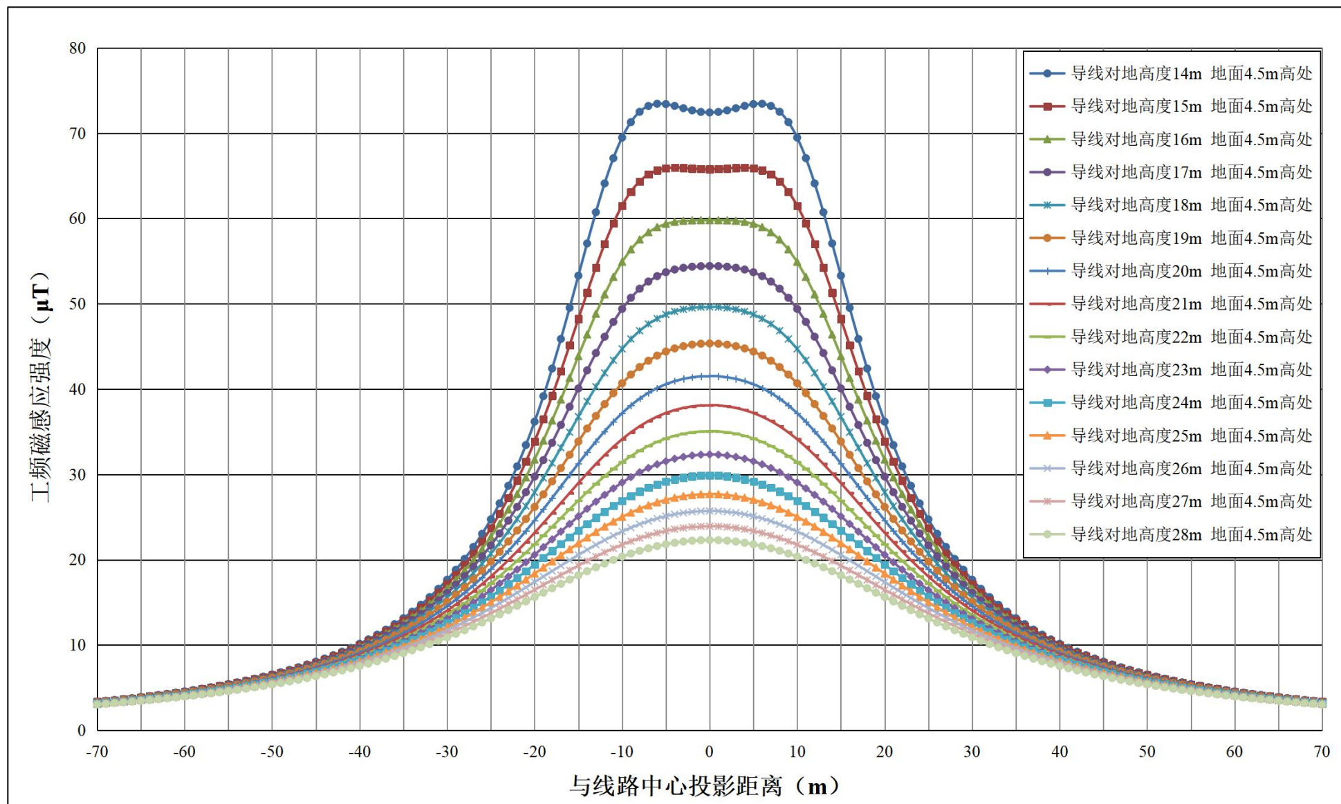
图 6.1-12 新建单回线路经过居民区时工频磁感应强度随距离变化趋势图 (距地面 4.5m 高处)
