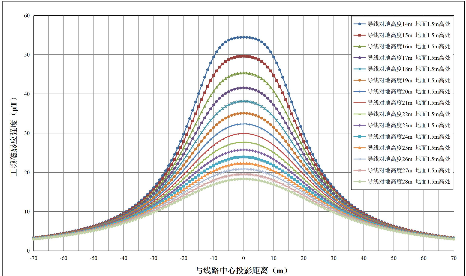
图 6.1-11 新建单回线路经过居民区时工频磁感应强度随距离变化趋势图 (距地面 1.5m 高处)
