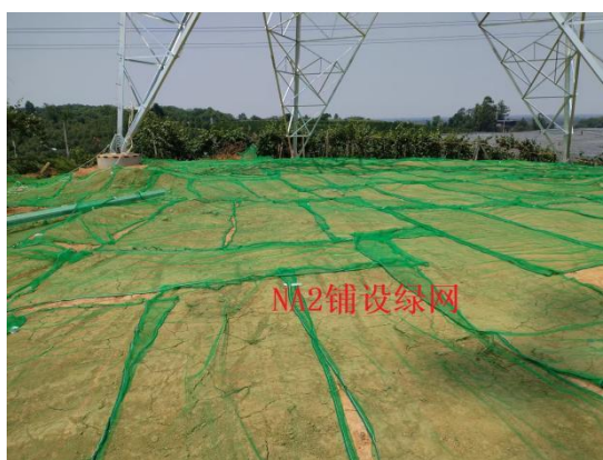
图8-2 塔基区铺设密目网
