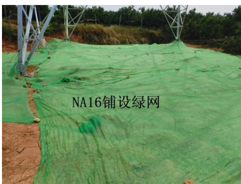
图8-2 塔基区铺设密目网
