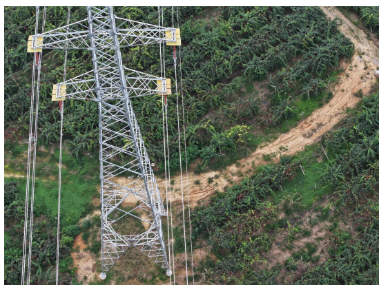
图5-3 NB4塔基存在侵蚀沟未回填
