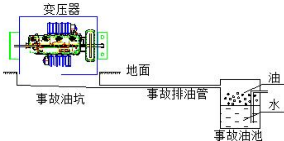
图 6-8 事故油池处理流程示意图
