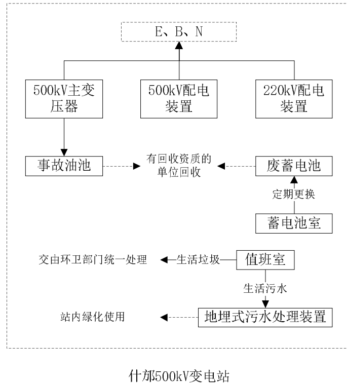
图 3-8 运行期工艺流程及产污环境图
