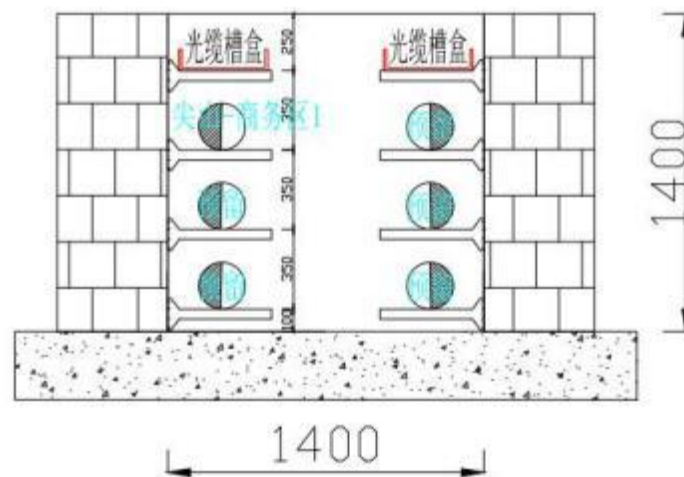
图 1.1-1 1.4\text{m} \times 1.4\text{m} 电缆沟敷设断面图
