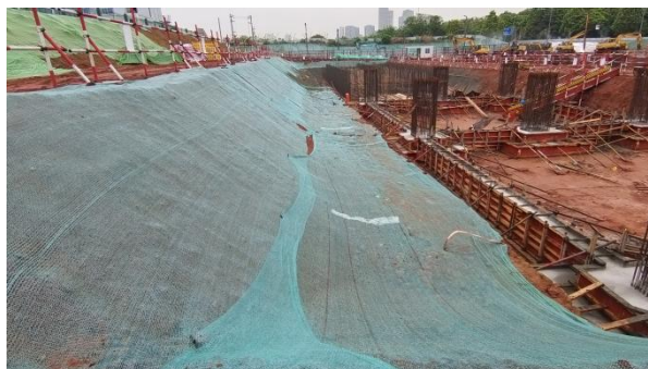
图8-4 基坑截水沟
