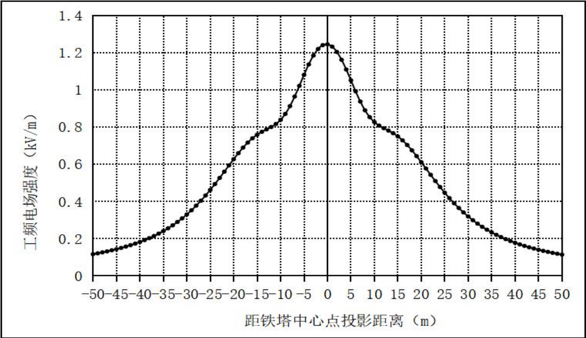
图 6-16 南天-海鑫一、二线 220kV 线路站外调整工程 导线最低离地高度 17.0m 时地面 1.5m 高处电场强度随距离变化图
