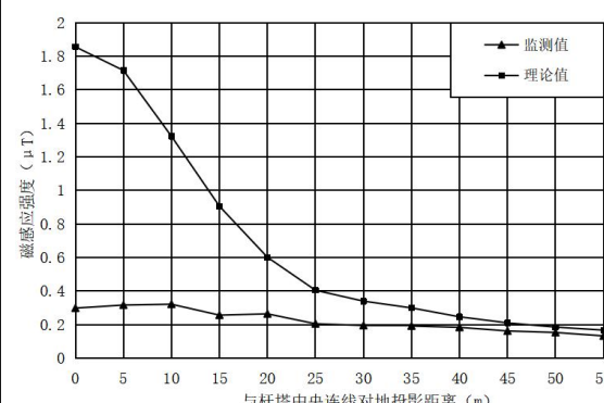
图 6-5 类比线路（220kV 江盘一二线） 磁感应强度随距中心线距离变化趋势图
