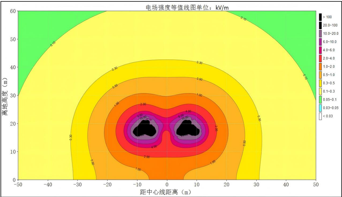
图 6-18 南天-海鑫一、二线 220kV 线路站外调整工程 导线最低离地高度 17.0m 时电场强度空间分布等值线图
