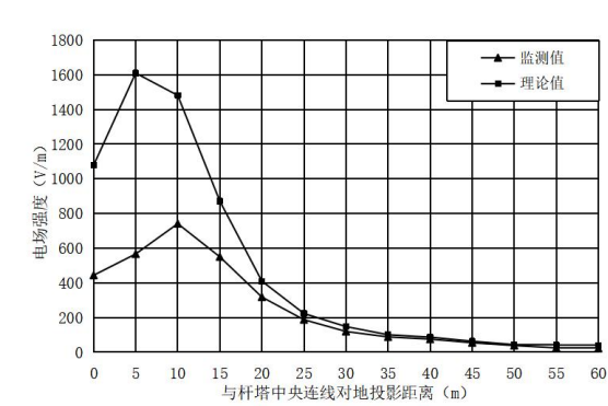
图 6-4 类比线路（220kV 江盘一二线） 电场强度随距中心线距离变化趋势图
