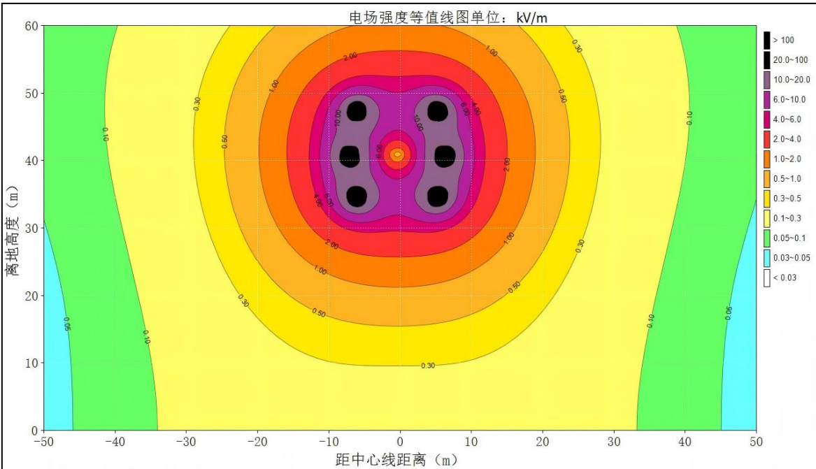
图 6-10 南天-圣达二线、南天-德胜 220kV 线路站外调整工程（新建双回段） 导线最低离地高度 34.5m 时电场强度空间分布等值线图
