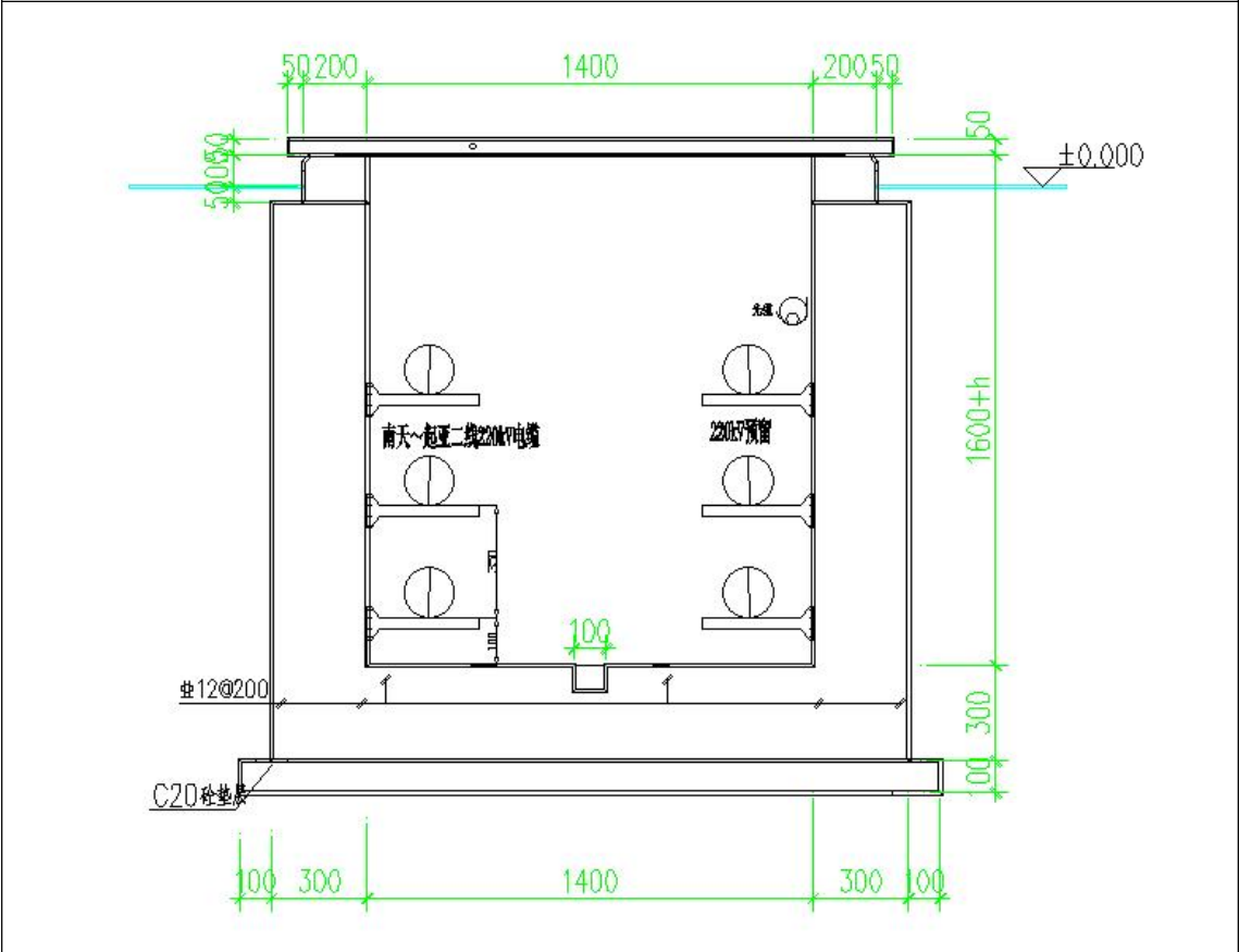
站内 1.4*1.3m 电缆沟电缆敷设断面示意图
