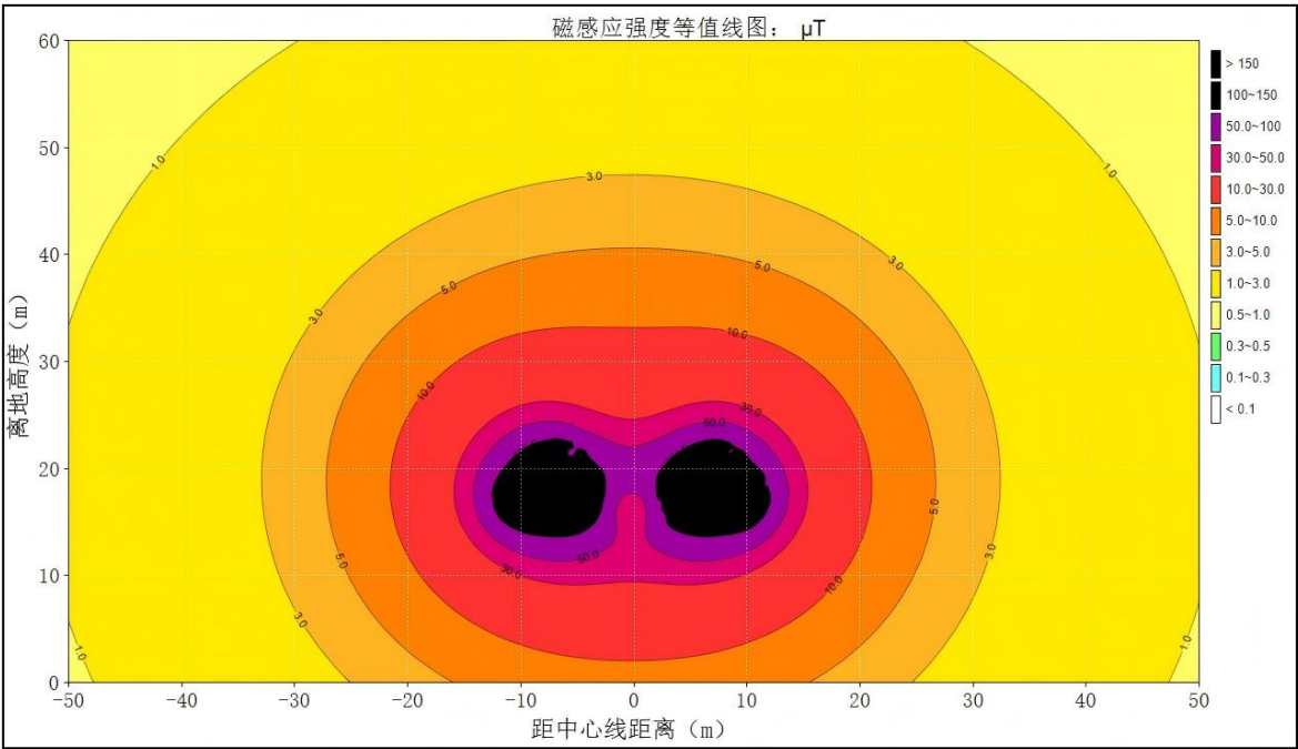
图 6-19 南天-海鑫一、二线 220kV 线路站外调整工程 导线最低离地高度 17.0m 时磁感应强度空间分布等值线图
