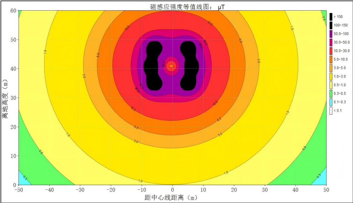
图 6-11 南天-圣达二线、南天-德胜 220kV 线路站外调整工程（新建双回段） 导线最低离地高度 34.5m 时磁感应强度空间分布等值线图
