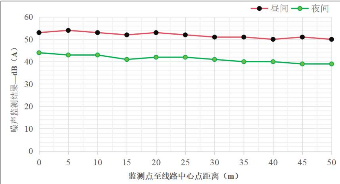
图 6-23 单回段类比线路 220kV 东泰线噪声随距中心线距离变化趋势图
