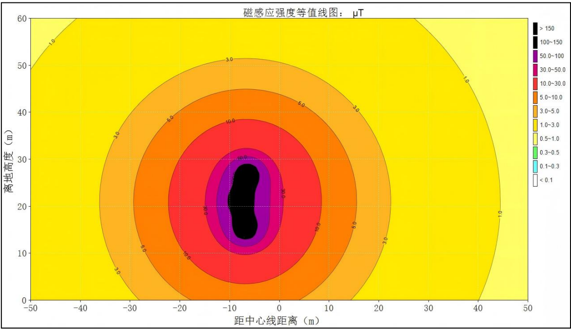
图 6-15 南天-圣达二线、南天-德胜 220kV 线路站外调整工程（新建单回段） 导线最低离地高度 15.0m 时磁感应强度空间分布等值线图
