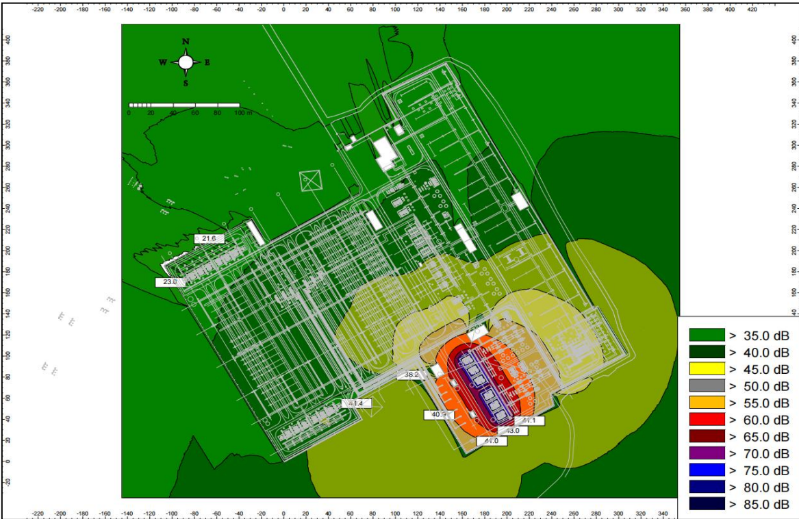
图 6-20 南天 500kV 变电站本次扩建后的噪声预测结果（有声屏障部分）
