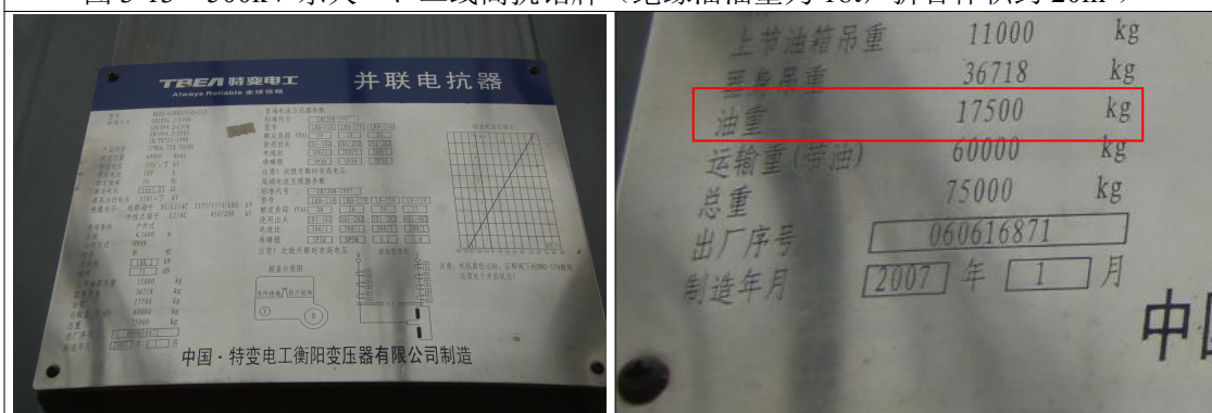
图 3-14 500kV 宁天线高抗铭牌（绝缘油油量为 17.5t，折合体积约 19.5m 3 ）
