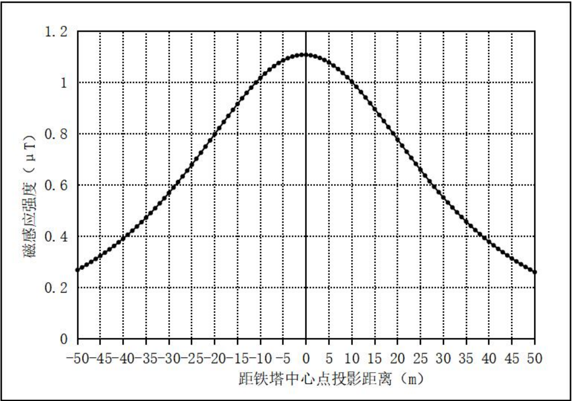
图 6-9 南天-圣达二线、南天-德胜 220kV 线路站外调整工程（新建双回段） 导线最低离地高度 34.5m 时地面 1.5m 高处工频磁场随距离变化图
