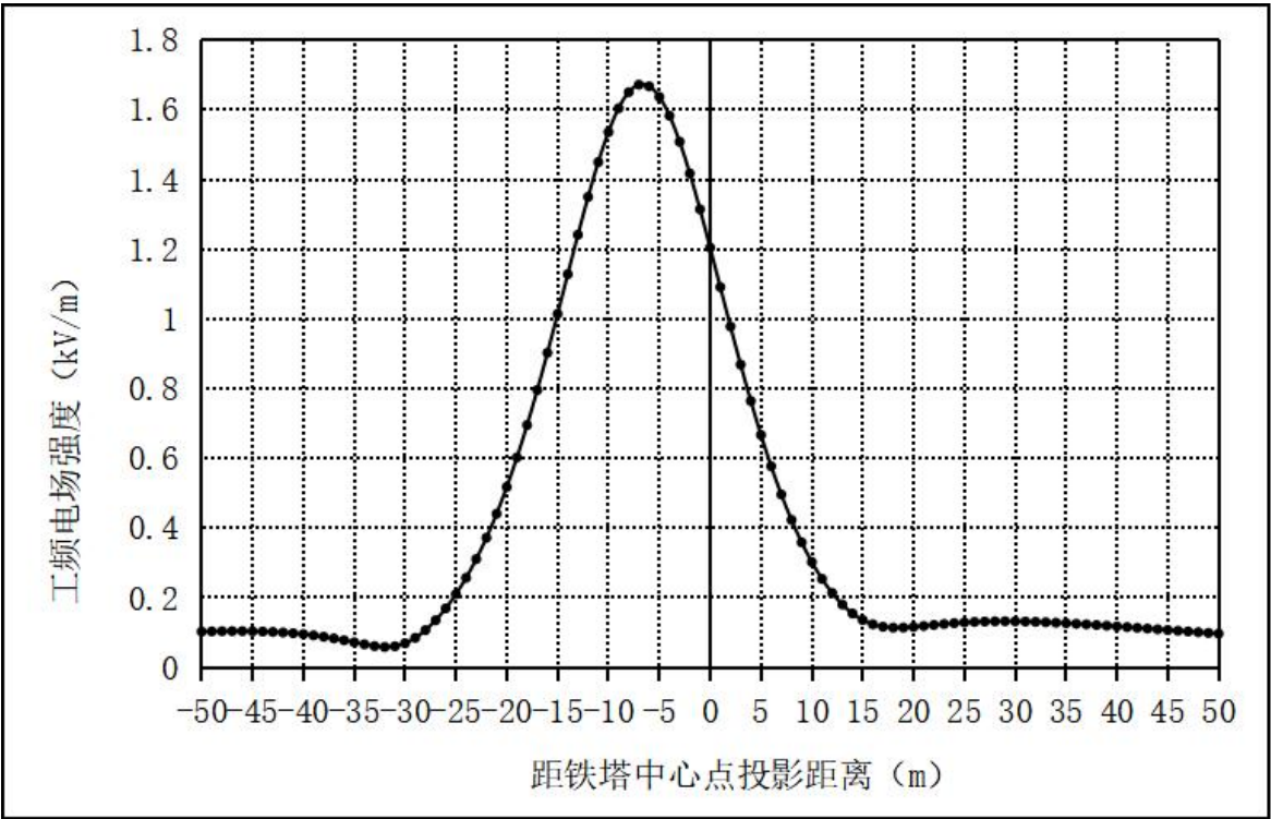
图 6-12 南天-圣达二线、南天-德胜 220kV 线路站外调整工程（新建单回段） 导线最低离地高度 15.0m 时地面 1.5m 高处电场强度随距离变化图
