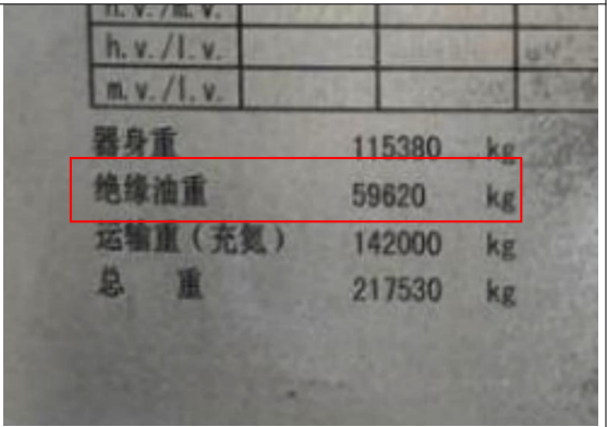
图 3-11 站内既有#1 主变铭牌（绝缘油油量为 59.62t，折合体积约 66.6m 3 ）
