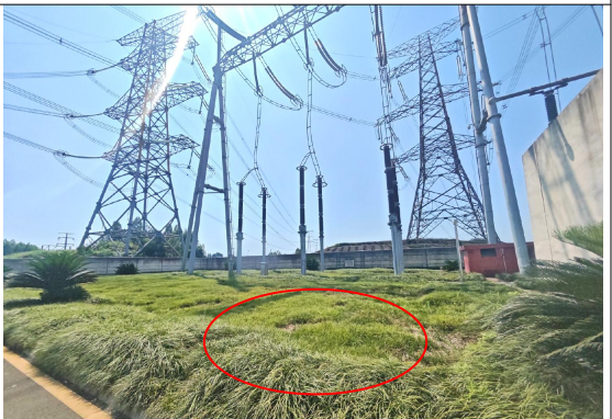
图 3-10 500kV 宁天线高抗事故油池（约 20m 3 ）
