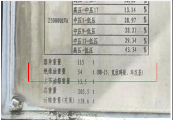
图 3-12 站内既有#2 主变铭牌（绝缘油油量为 54t，折合体积约 60.3m 3 ）
