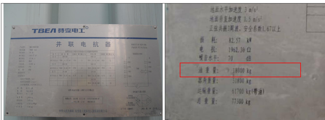
图 3-13 500kV 东天一、二线高抗铭牌（绝缘油油量为 18t，折合体积约 20m 3 ）
