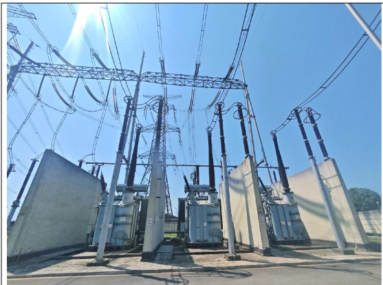
图 3-7 500kV 宁天线高抗、各相之间防火墙、各相下方事故油坑（约 10m 3 ）
