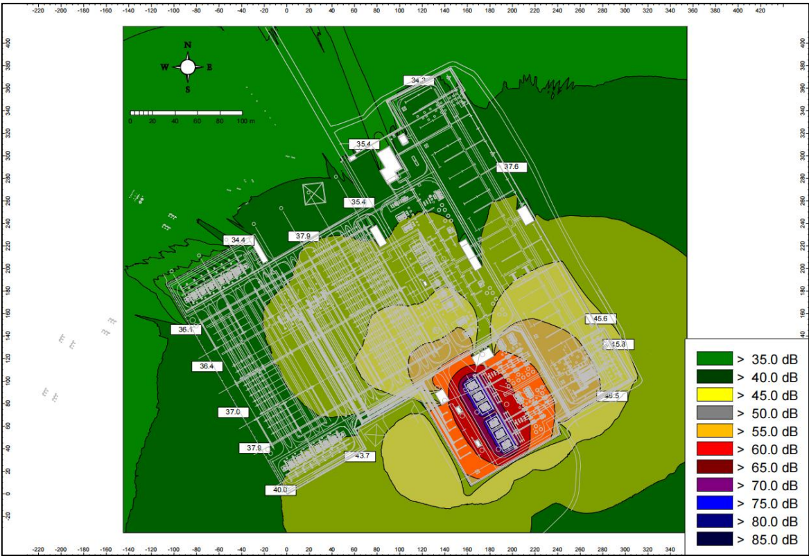
图 6-21 南天 500kV 变电站本次扩建后的噪声预测结果（无声屏障部分）
