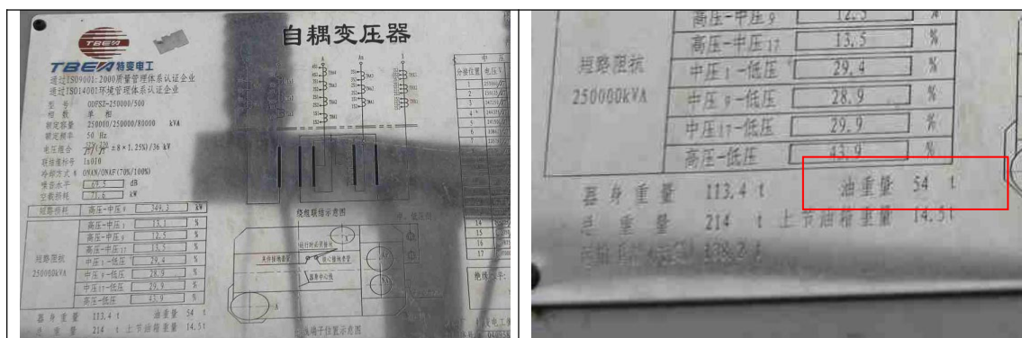
图 3-17 本次新增#3 主变铭牌 (利用谭家湾 500kV 变电站#1 主变, 绝缘油油量为 54t, 折合体积约 60.3m 3 )
