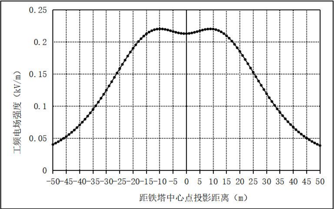
图 6-8 南天-圣达二线、南天-德胜 220kV 线路站外调整工程（新建双回段） 导线最低离地高度 34.5m 时地面 1.5m 高处电场强度随距离变化图
