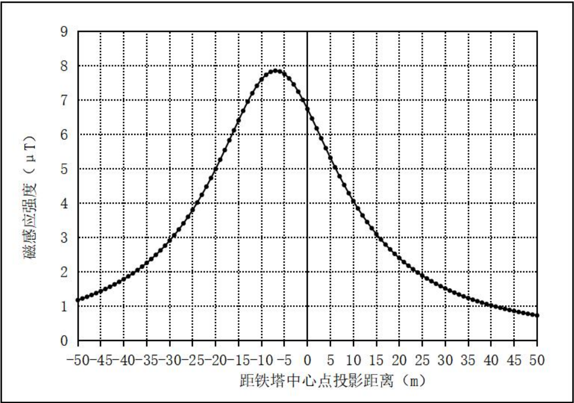
图 6-13 南天-圣达二线、南天-德胜 220kV 线路站外调整工程（新建单回段） 导线最低离地高度 15.0m 时地面 1.5m 高处工频磁场随距离变化图
