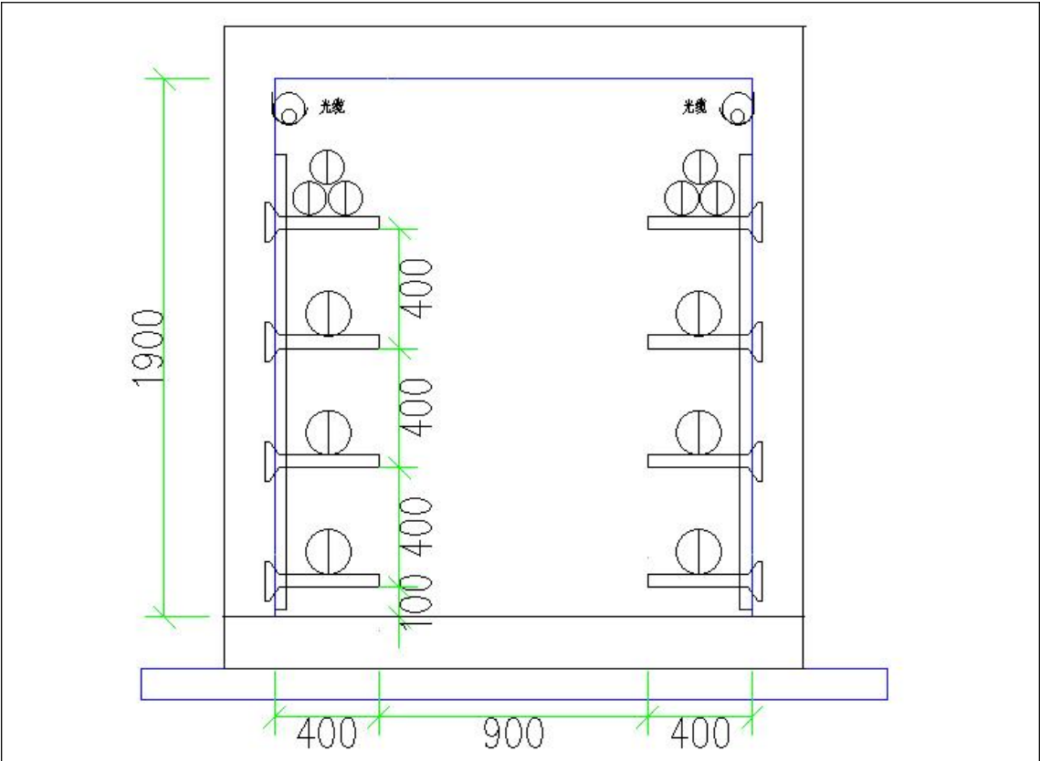
新建 1.7*1.9m 电缆沟电缆敷设断面示意图
