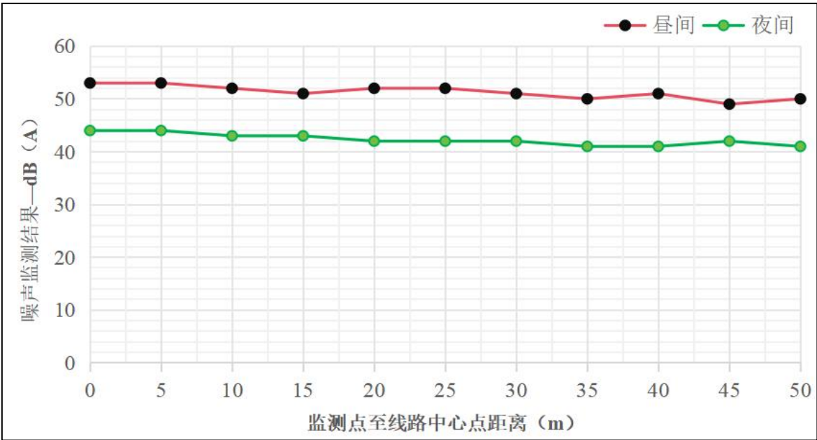
图 6-22 双回段类比线路 220kV 江盘一二线噪声随距中心线距离变化趋势图
