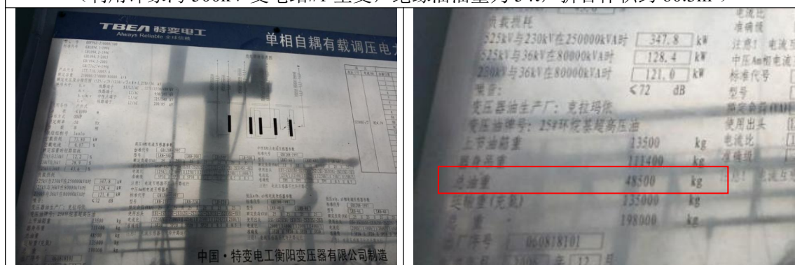
图 3-18 本次新增#4 主变铭牌 (利用谭家湾 500kV 变电站#2 主变, 绝缘油油量为 48.5t, 折合体积约 54.2m 3 )
