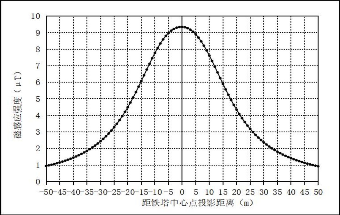
图 6-17 南天-海鑫一、二线 220kV 线路站外调整工程 导线最低离地高度 17.0m 时地面 1.5m 高处工频磁场随距离变化图
