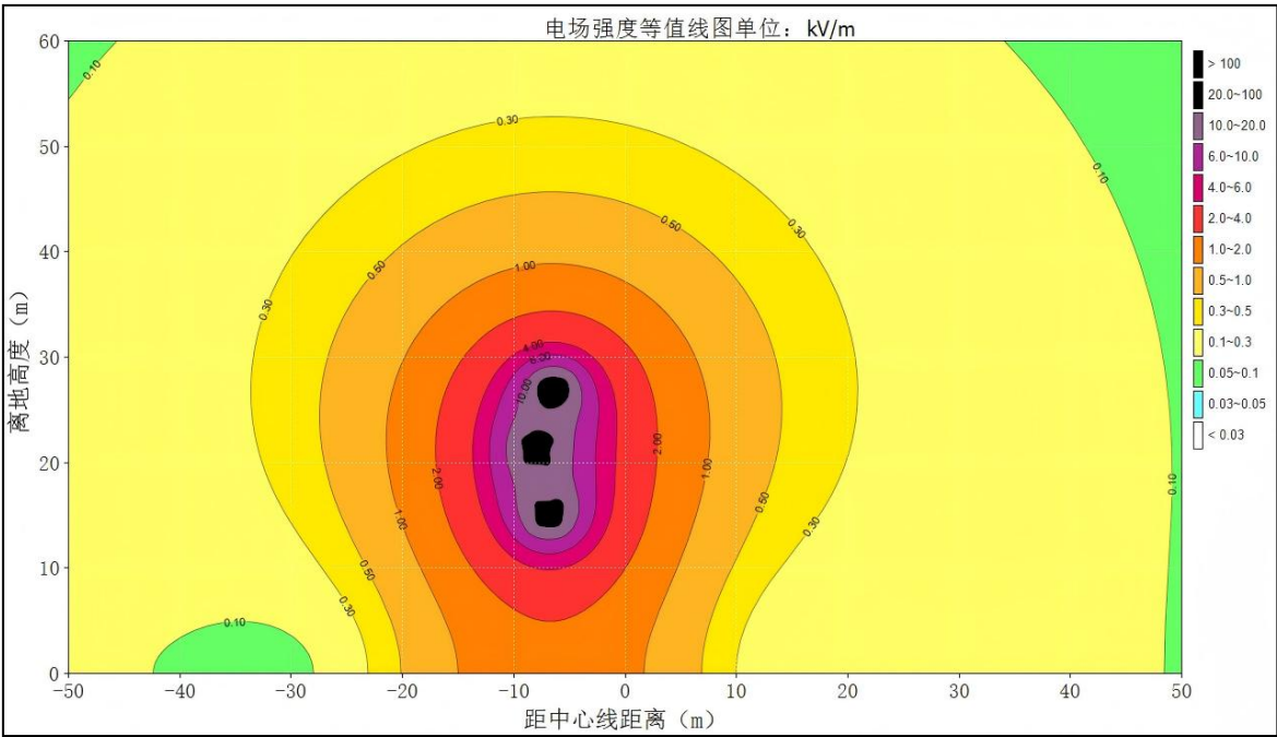
图 6-14 南天-圣达二线、南天-德胜 220kV 线路站外调整工程（新建单回段） 导线最低离地高度 15.0m 时电场强度空间分布等值线图
