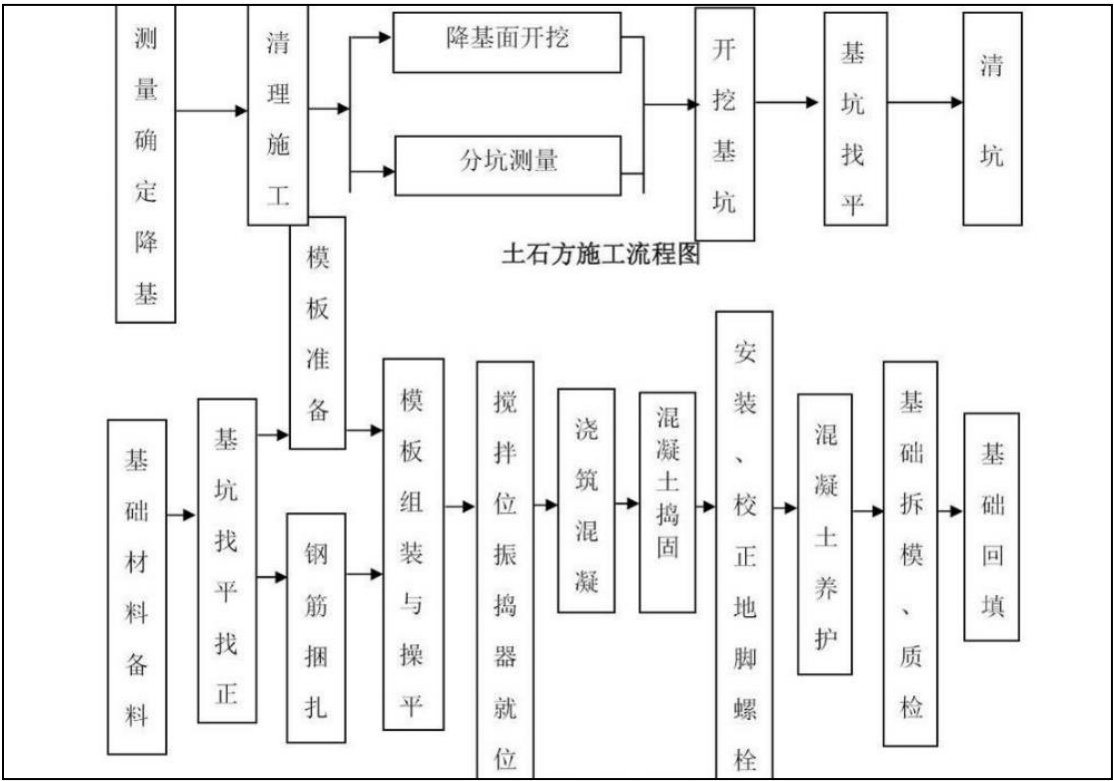
图 3-16 塔基基础施工工艺流程图
